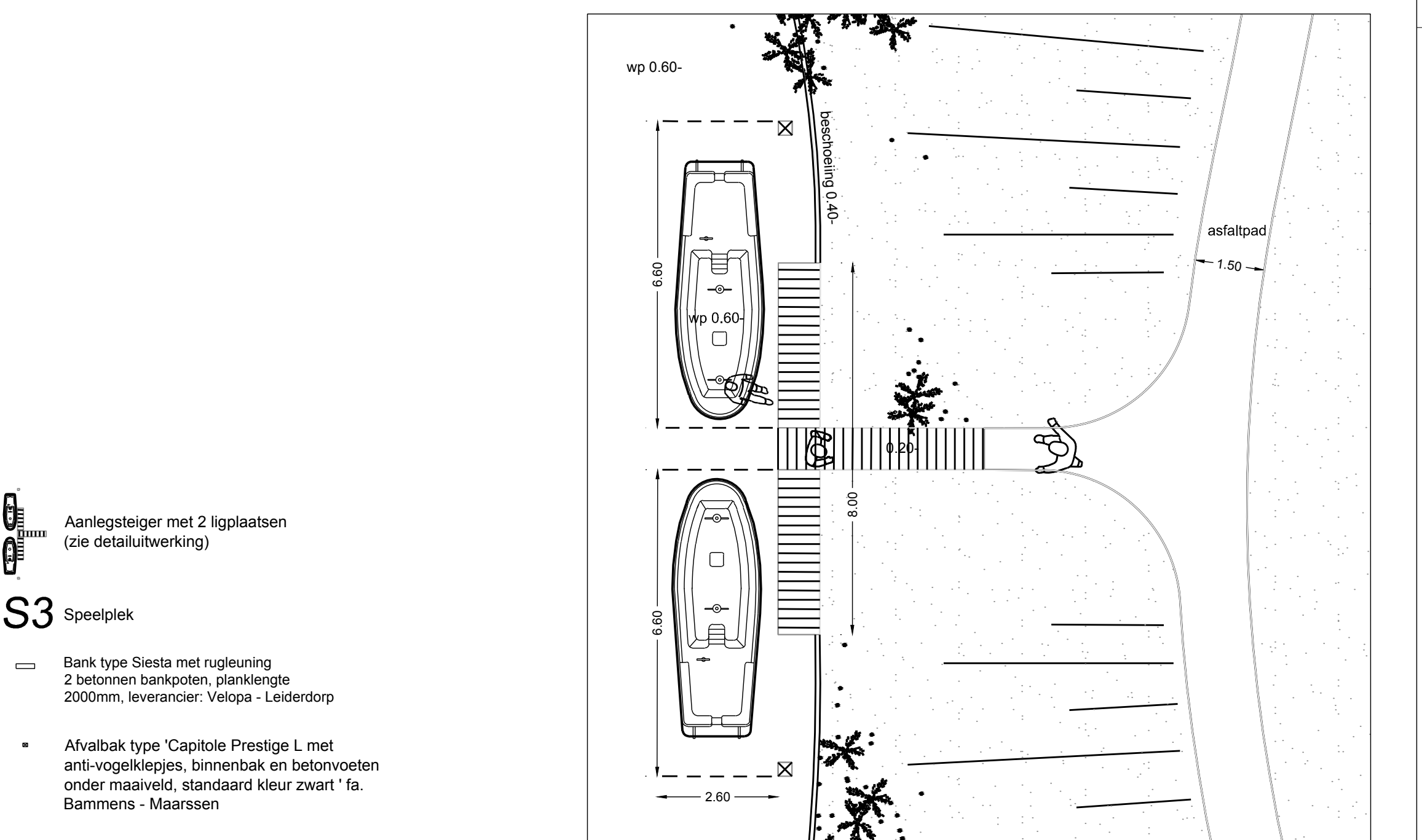
Uitwerking aanlegsteiger - schaal 1:100
