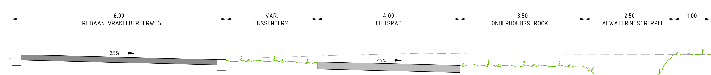
DWARSPROFIEL 4 SCHAAL 150
