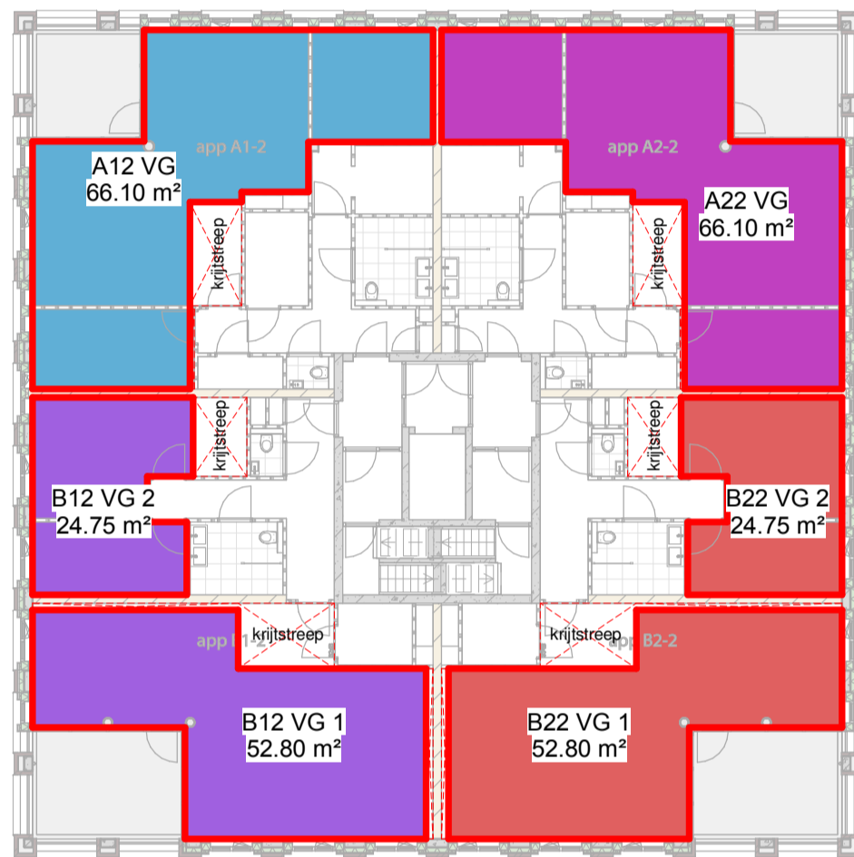
02 tweede verdieping
