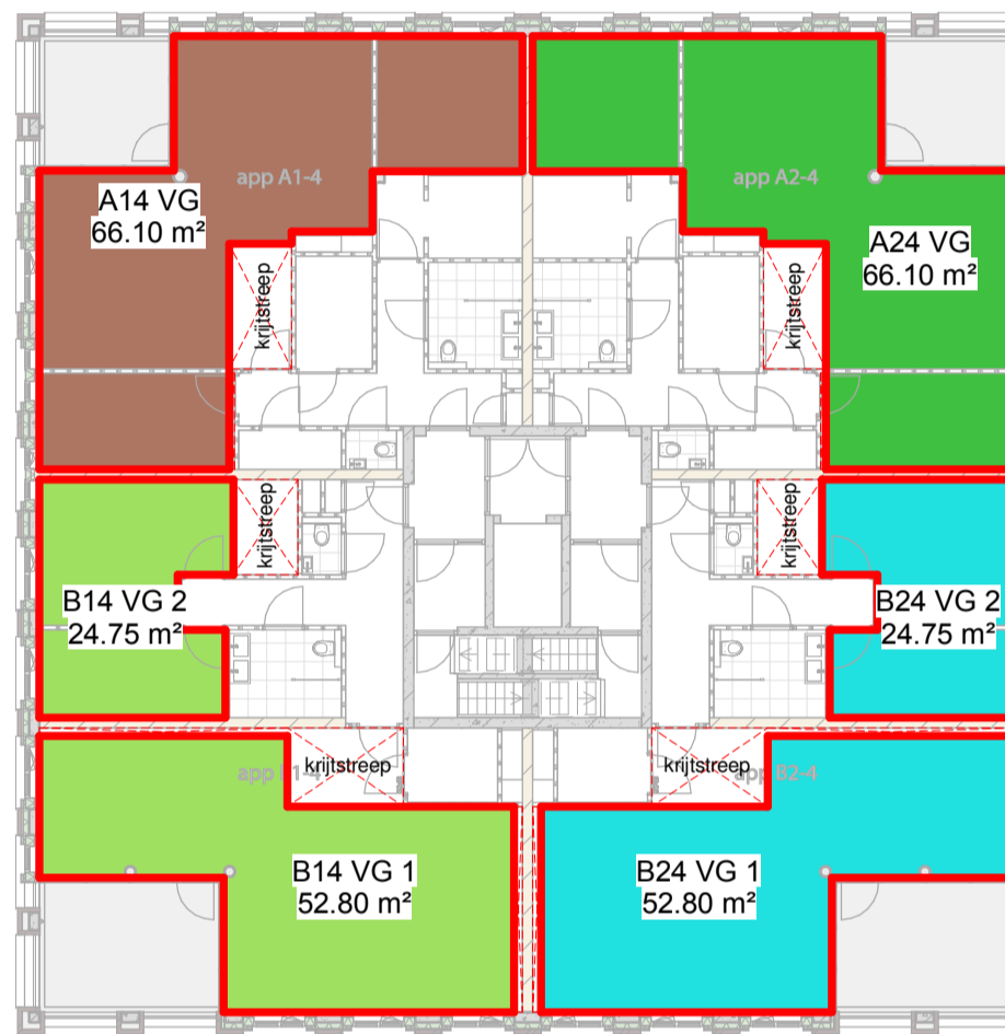
04 vierde verdieping
