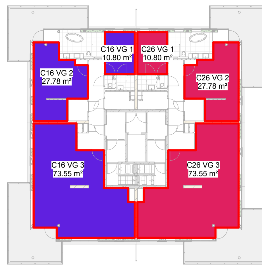
06 zesde verdieping
