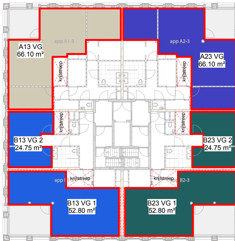
03 derde verdieping
