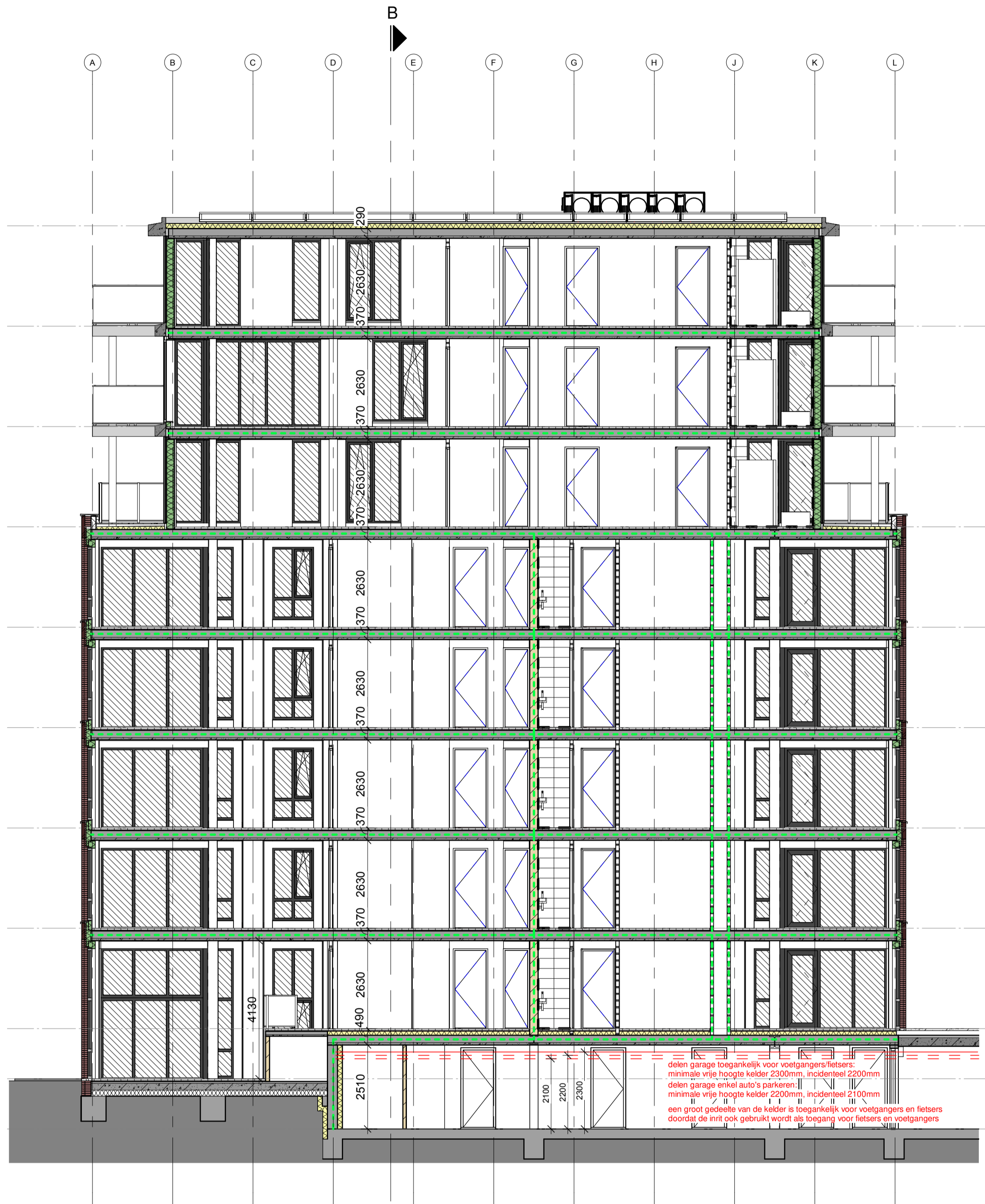
doorsnede A-A 1 : 100
