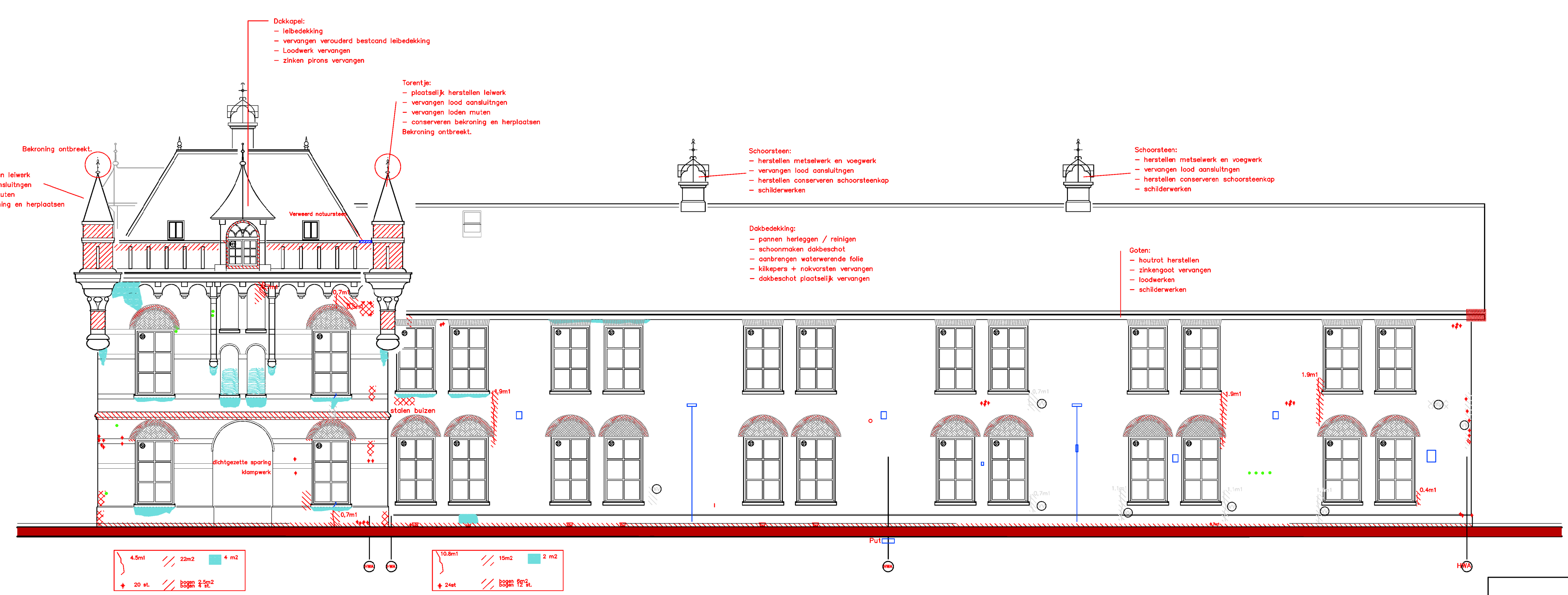
Vleugel 4 Noordzijde
