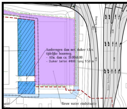
Water eindsituatie (paars) en bouwsituatie (blauw)
