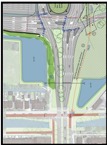
Water KKC eindsituatie
