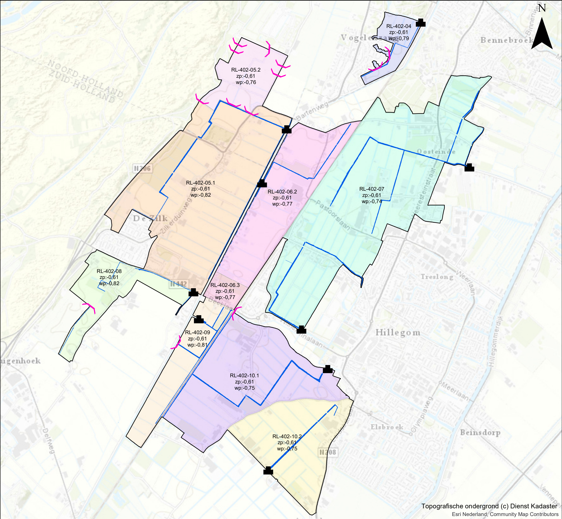
Kaart 9a: Peilvoorstel Peilvakken De Zilk
