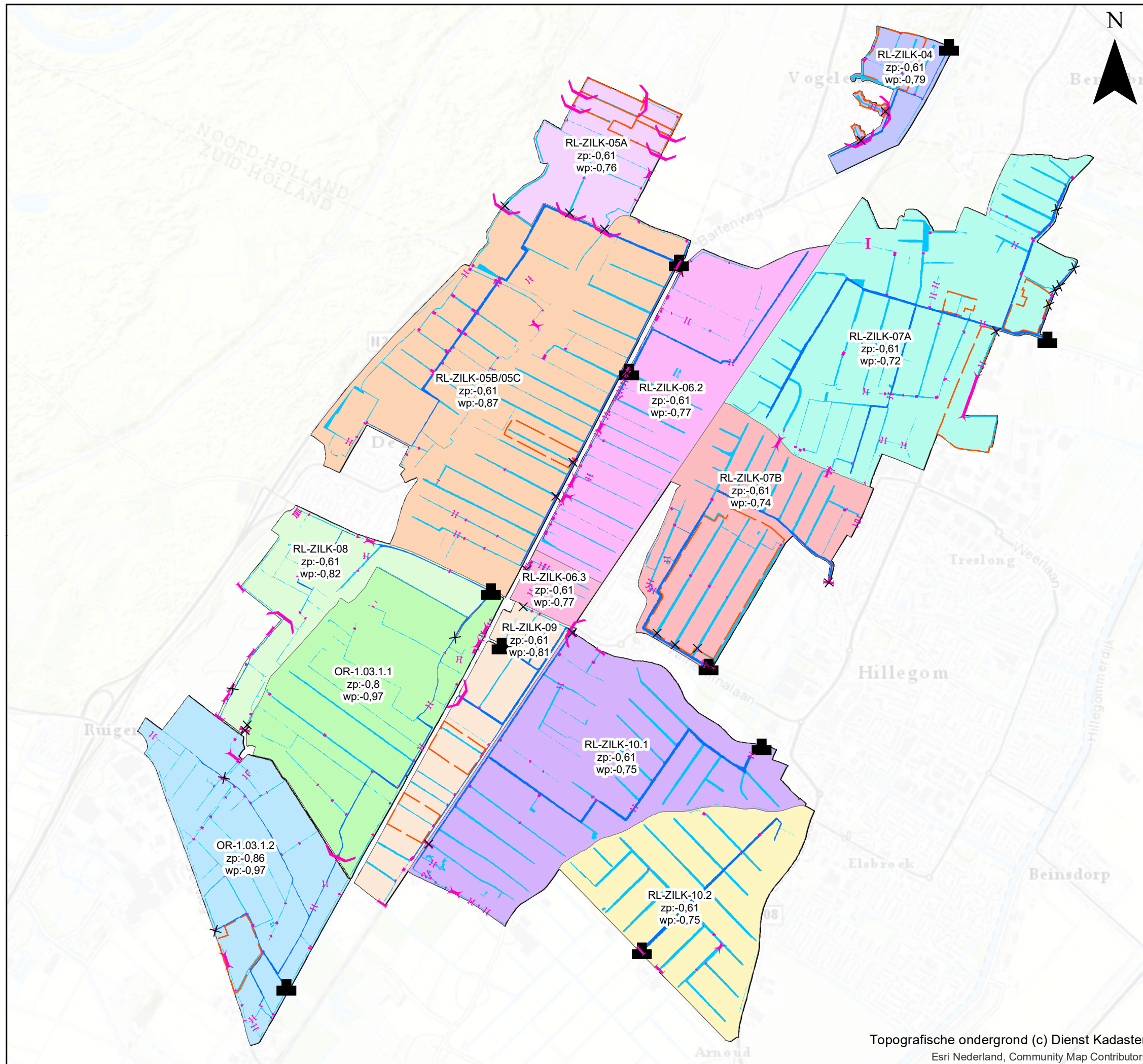
Kaart 6: Huidige waterhuishoudkundige situatie (o.b.v. praktijkpeilen)
