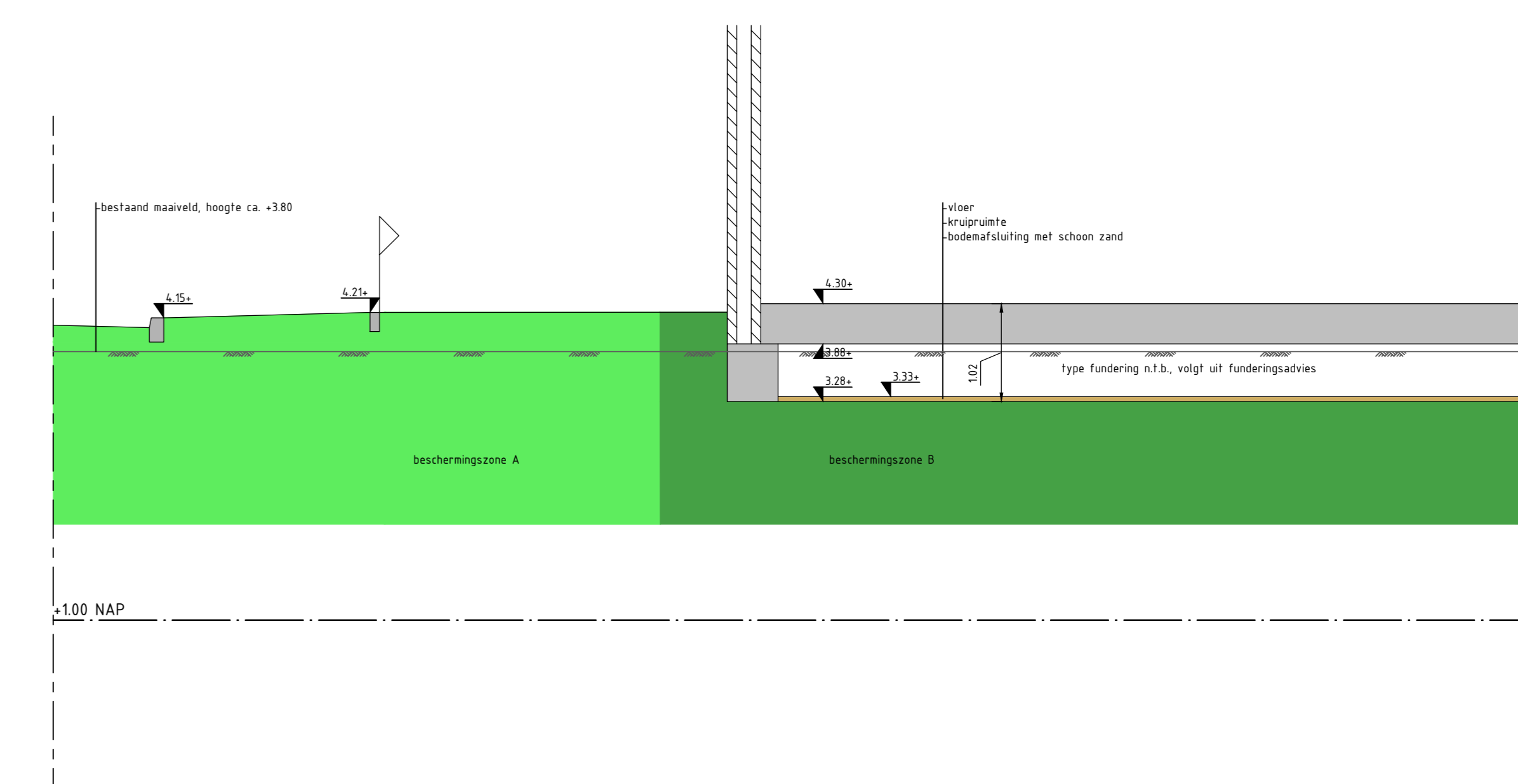
Doorsnede A-A Schaal 1:50
