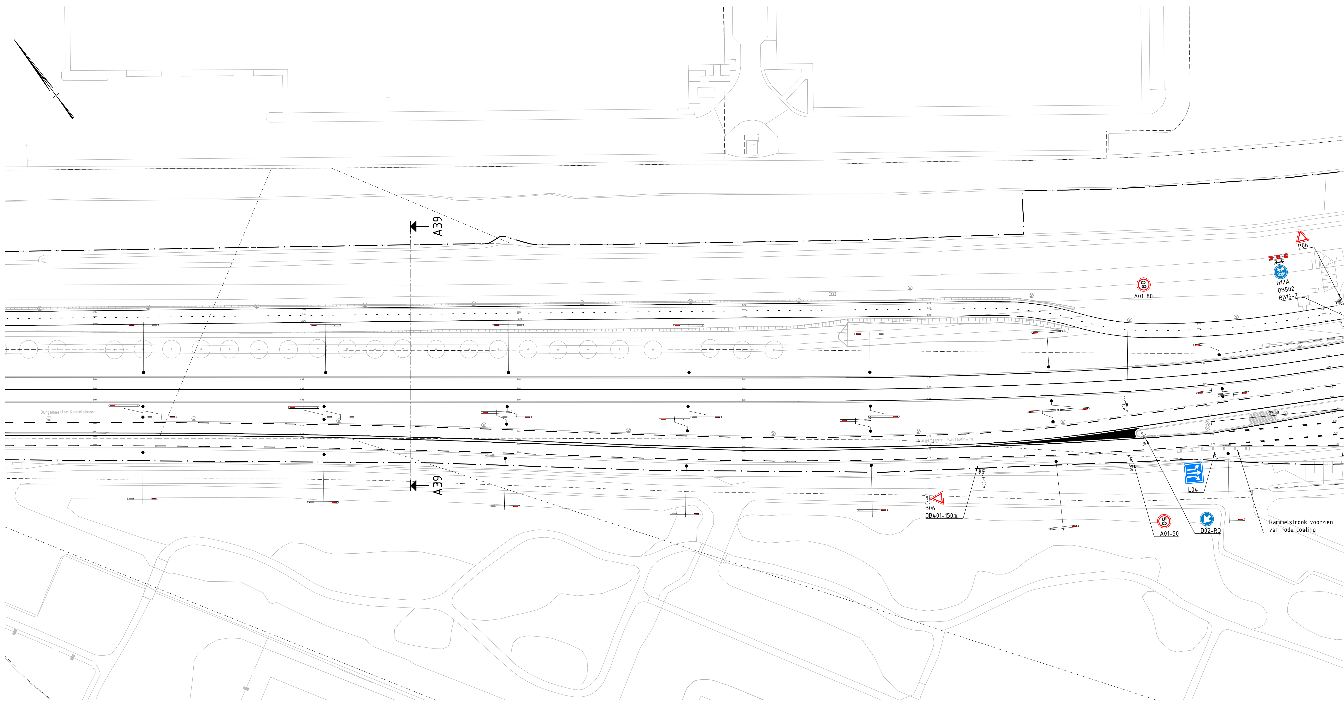
Overzicht 08.02 Schaal 1:500
