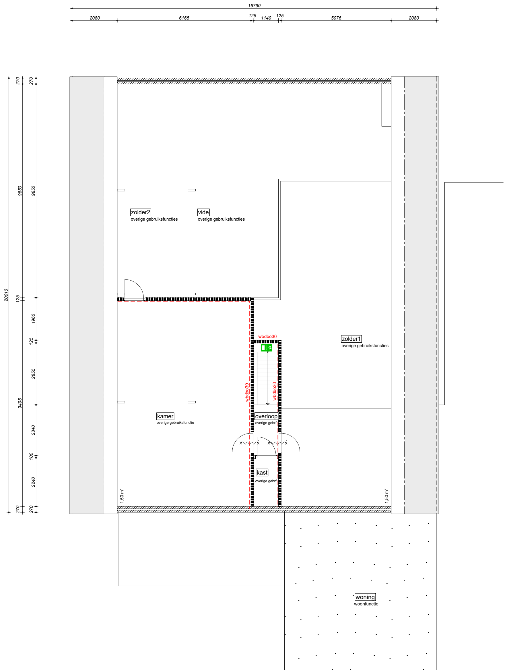
PLATTEGROND VERDIEPING
