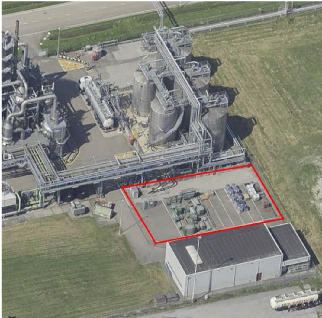
Figuur 2: overzichtsfoto. Links de bestaande fabriek, rechts boven het bestaande tankput, rood omlijnt de locatie voor de nieuwe tanks.
