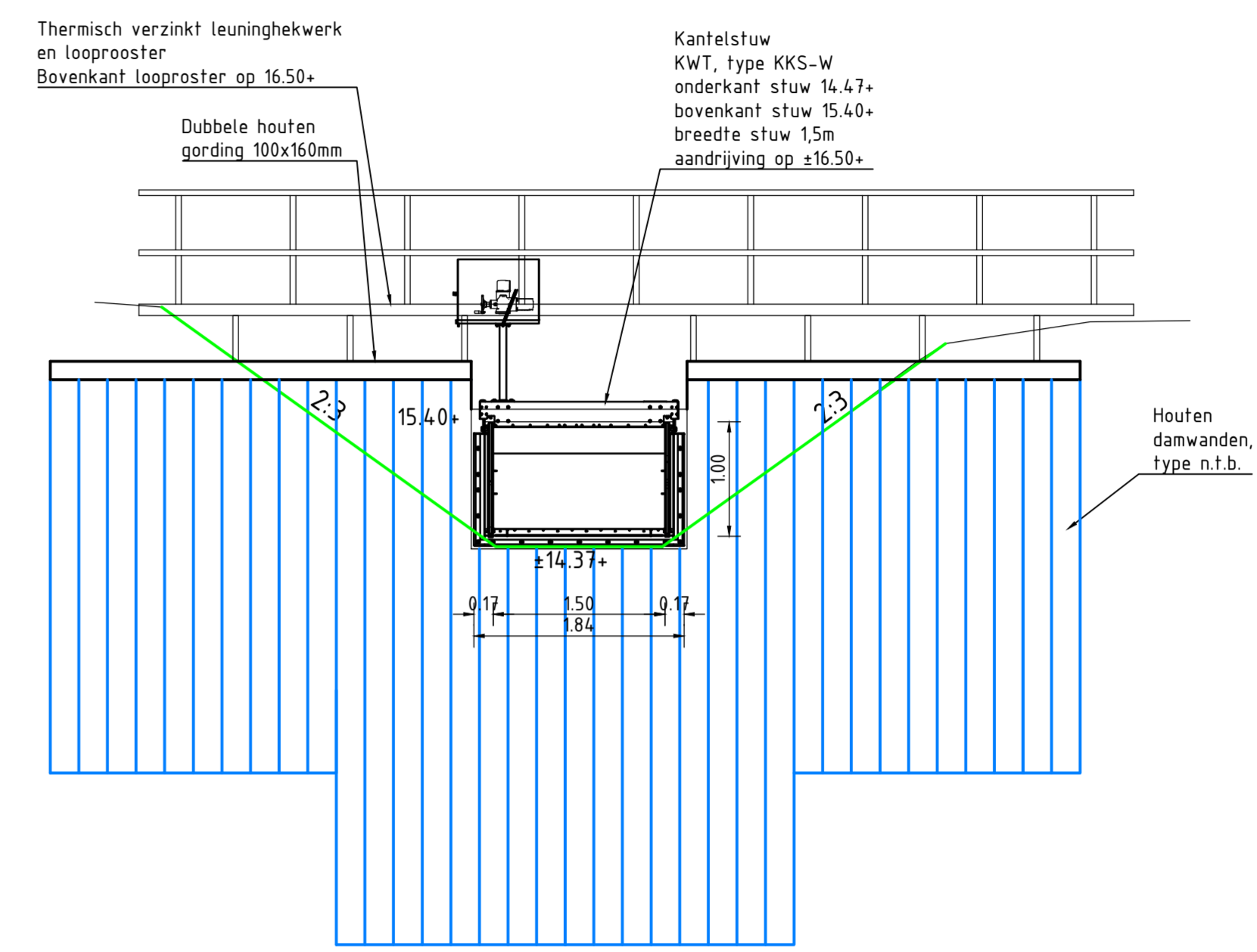
VOORAANZICHT STUW 2 schaal 1:50
