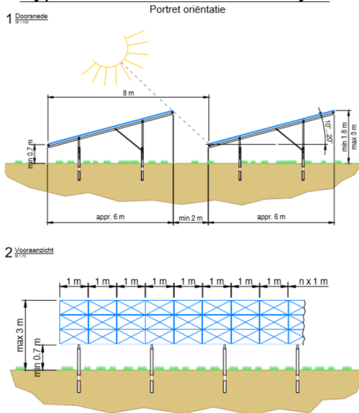
Figuur 3. Situatietekening positie zonnepanelen en ruimte tussen de paden. Bron: IB VOGT GmbH, 2020
