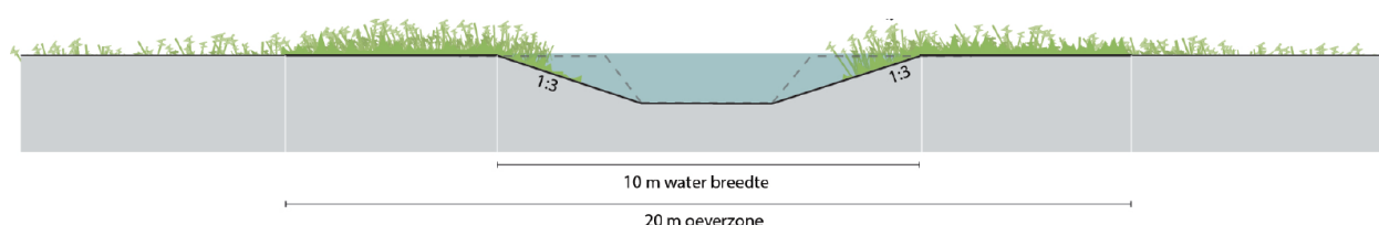
Figuur 47. Dwarsprofiel verbrede sloot (20 m 2 ) in kraggenlandschap
