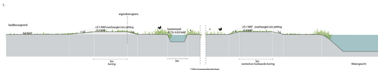
Figuur 58. Dwarsprofiel kering en Tautenburger Sloop
