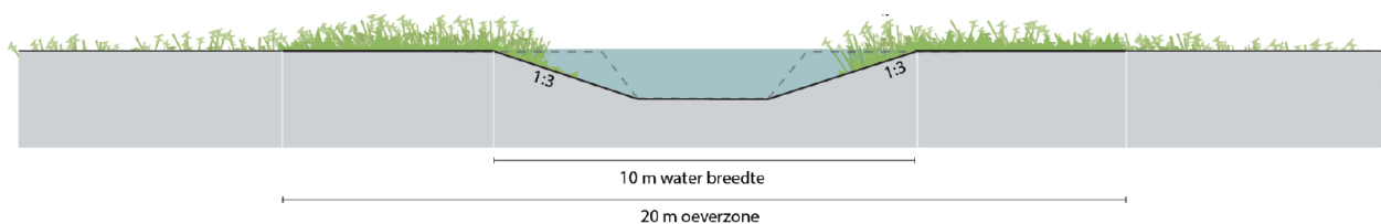
Figuur 40. Dwarsprofiel verbrede sloot (10 m 2 ) in kraggenlandschap
