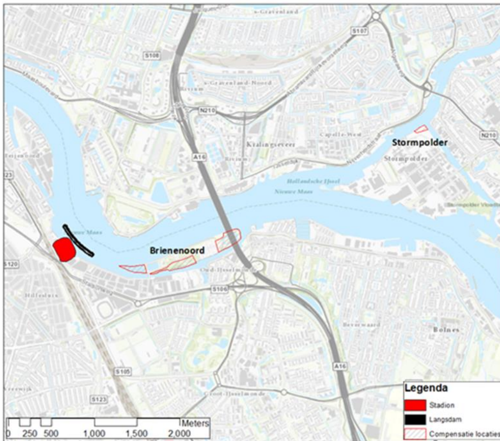
Figuur 2. Waterbergingscompensatielocaties (Stormpolder en Eiland van Briene Noord), waarvan Stormpolder wordt gebruikt voor ecologische vereffening van negatieve effecten. Ook aangegeven zijn de ingrepen (stadion en langsdam), waarvan de langsdam (inclusief het luwe gebied daarachter) door een goede inrichting bijdraagt aan de ecologische vereffening
