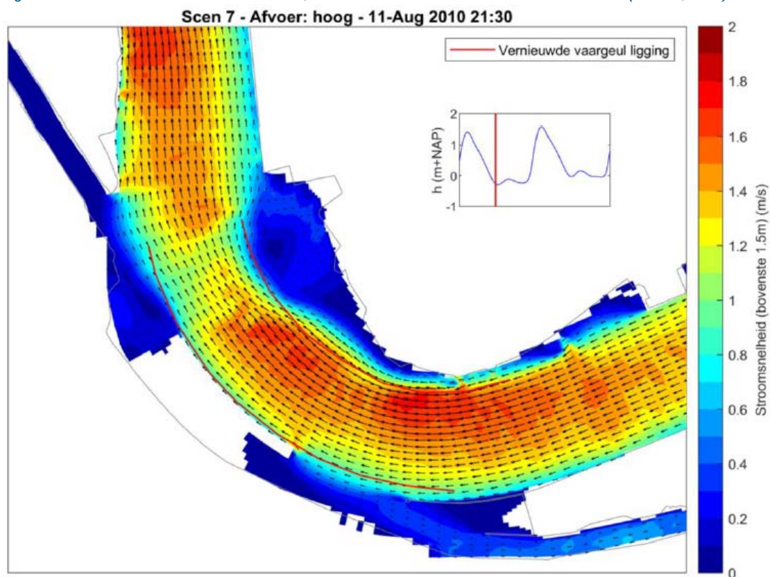
Figuur 20: Ebstroomsnelheid in de bovenste 1,5m van de waterkolom voor de eindsituatie (Svasek, 2020).
