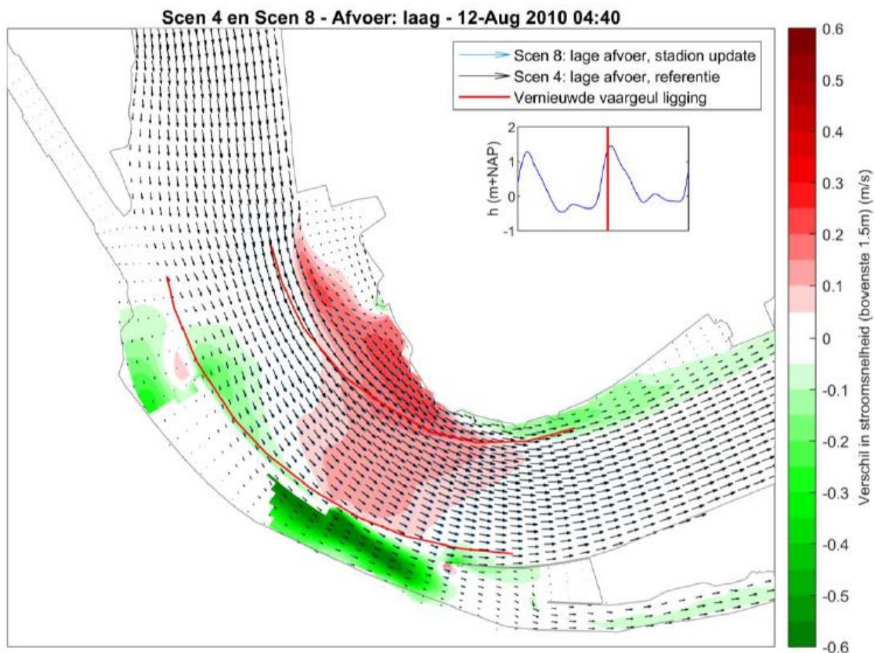
Figuur 24: Verschil in stroomsnelheden tussen de referentie- en eindsituatie voor maximale vloed-storm voor de bovenste 1,5 meter van de waterkolom (Svasek, 2020).
