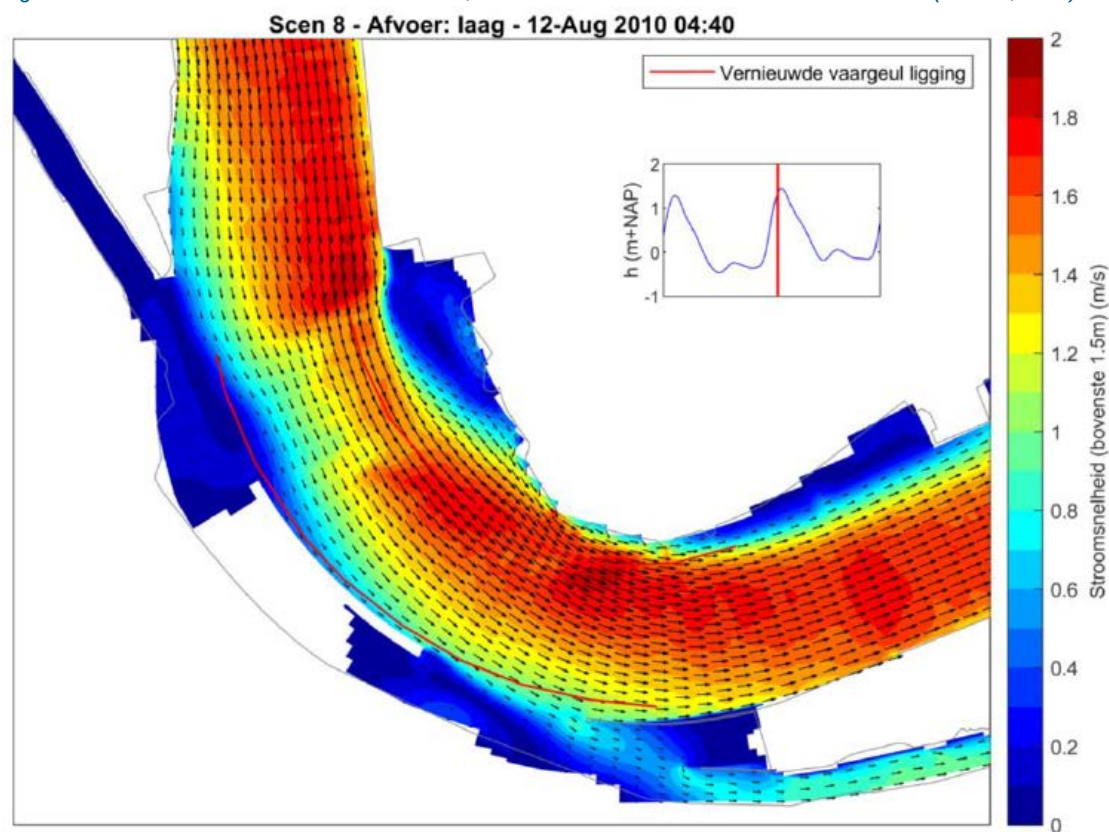
Figuur 23: Vloedstroomsnelheid in de bovenste 1,5m van de waterkolom voor de eindsituatie (Svasek, 2020).
