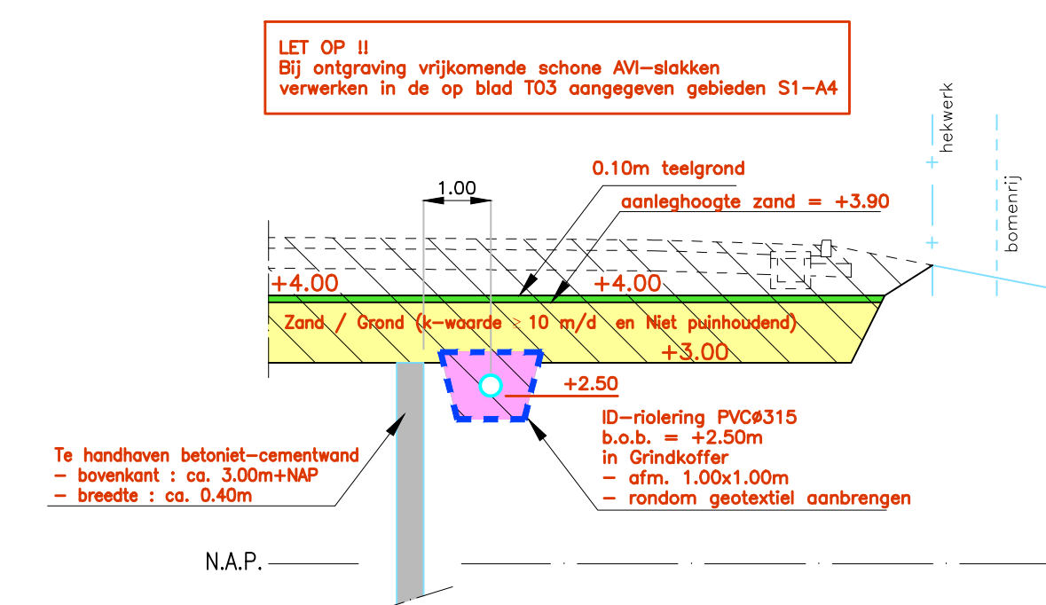
Profiel 6-6 schaal 1:100
