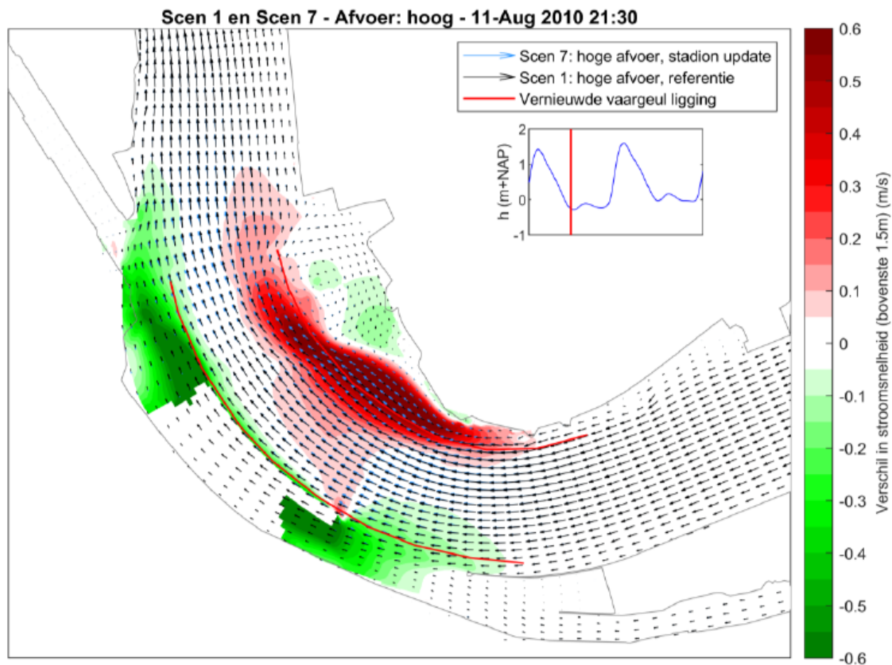
Figuur 21: Verschil in stroomsnelheden tussen referentie- en eindsituatie tijdens maximale ebstroom voor de bovenste 1,5 meter van de waterkolom (Svasek, 2020).
