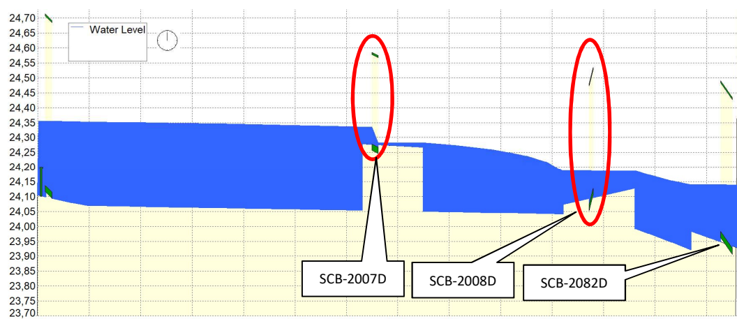
Figuur 2-10: Verloop bodemprofiel watergang Schelkensbeek tot Meerlebroek – 0,5 MA
