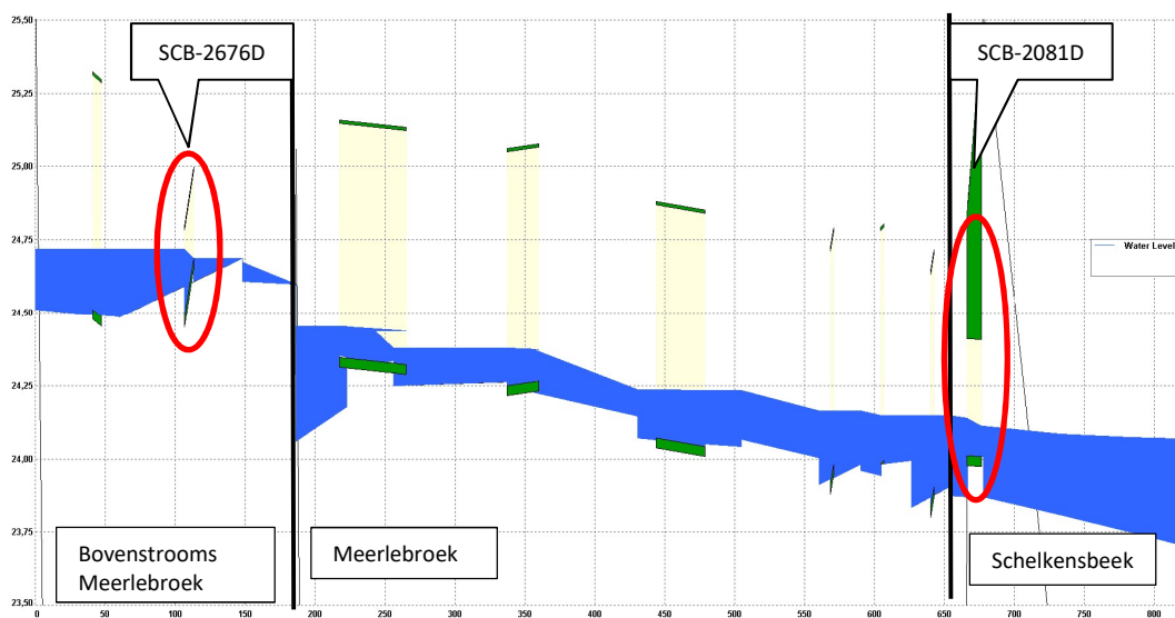
Figuur 2-6: Verloop bodemprofiel Meerlebroek, met in de rode cirkels de te vervangen duikers, waarvan de duiker in de Schelkensbeek staat beschreven in paragraaf 2.6 – 0,5 MA
