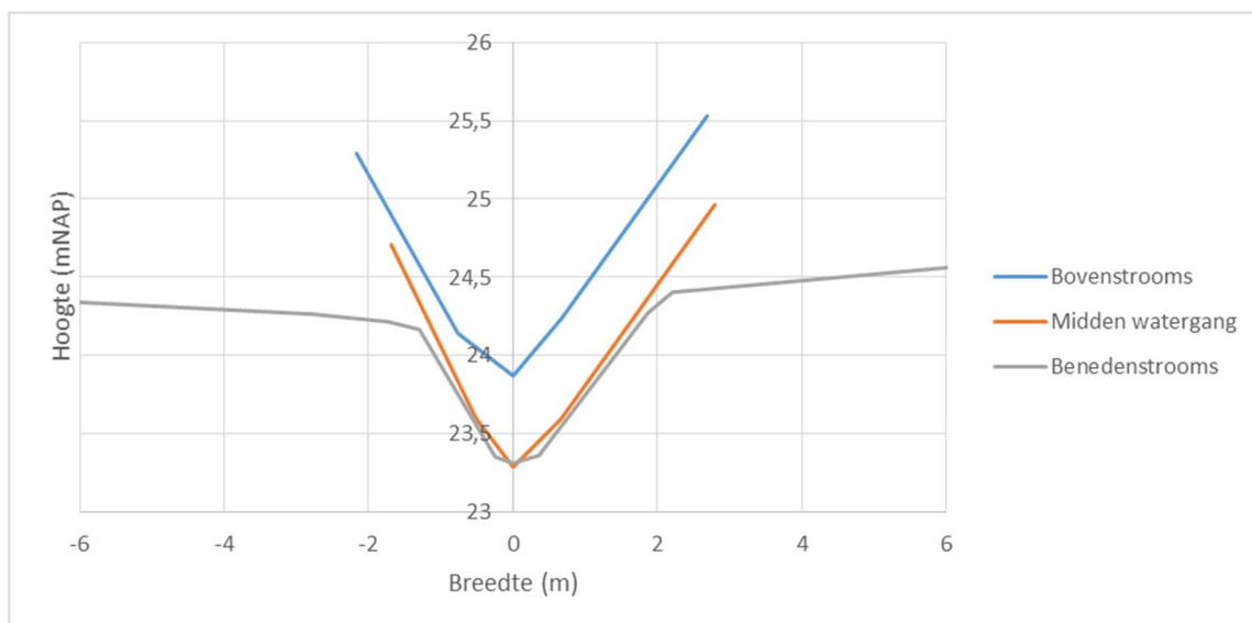
Figuur 2-14: Huidige profielen watergang Schelkensbeek, bovenstrooms is profiel H, profiel in midden van watergang is I, benedenstrooms is profiel J (zie bijlage 2)
