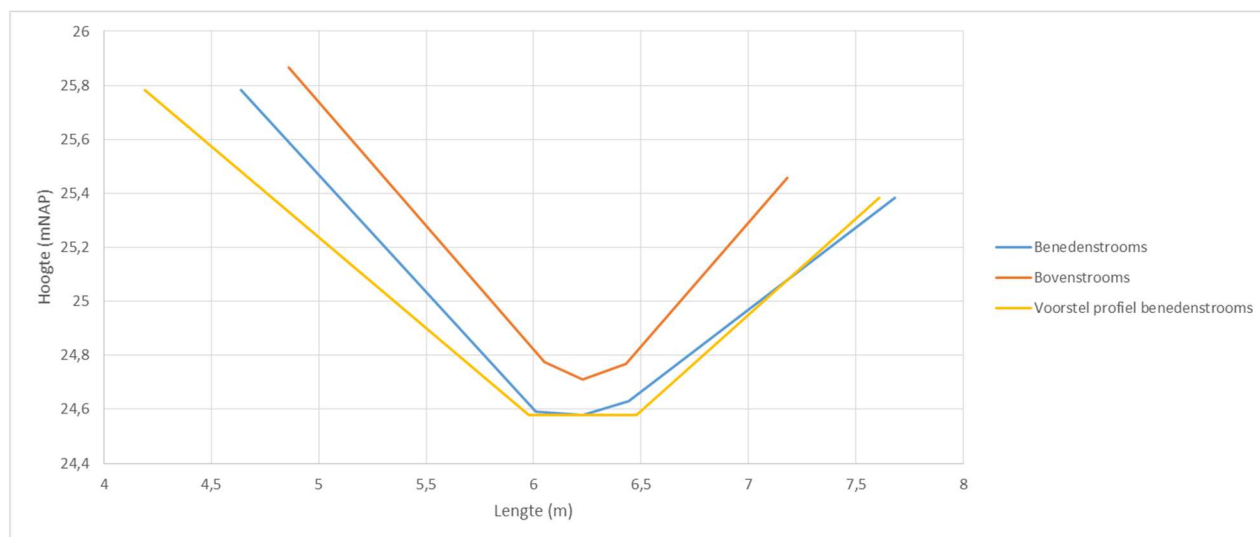
Figuur 2-5: Huidige profielen Sint Lambertusbeek, bovenstrooms is profiel A, benedenstrooms is profiel B (zie bijlage 2)
