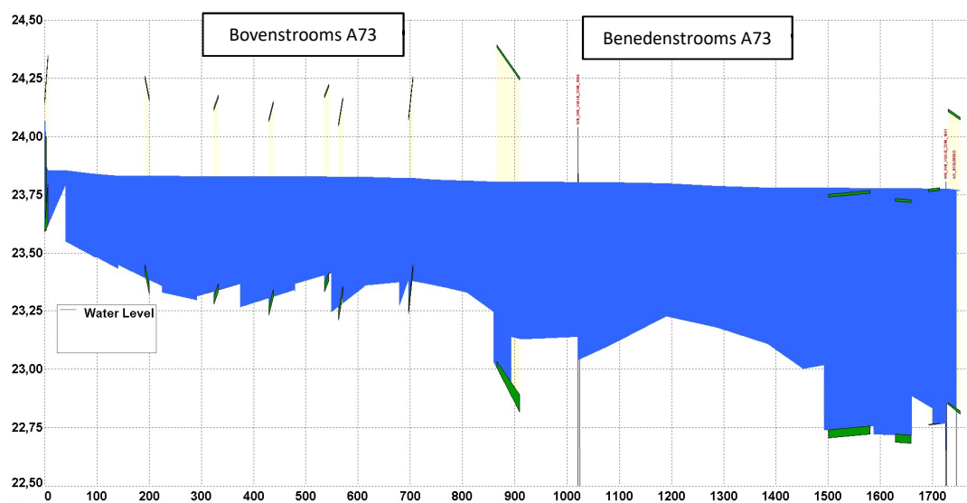
Figuur 2-13: Bodemverloop Schelkensbeek boven- en benedenstrooms A73.
