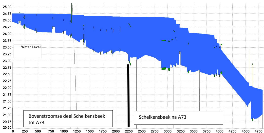
Figuur 2-1: Modelberekening en situatieschets van waterproblematiek bovenstroomse deel Schelkensbeek van de T100 winterbui exclusief klimaattoeslag (huidige situatie).
