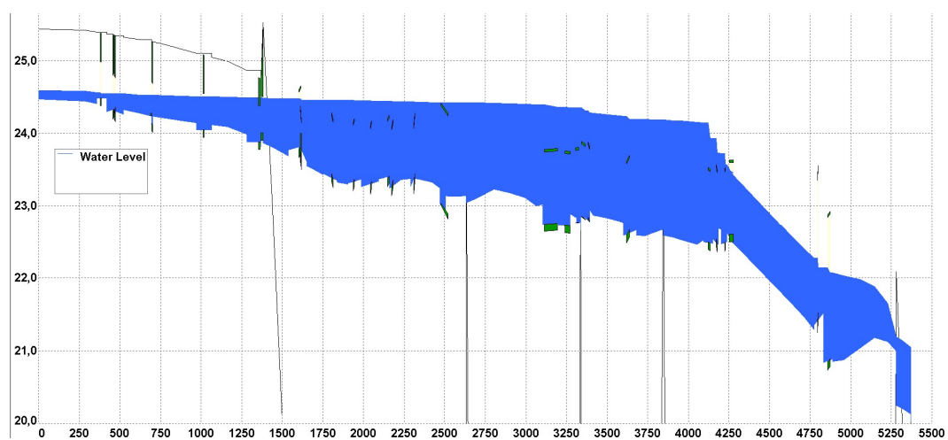
Figuur 2-2: Modelberekening en situatieschets van waterproblematiek bovenstroomse deel Schelkensbeek van de T25 winterbui exclusief klimaattoeslag (huidige situatie).
