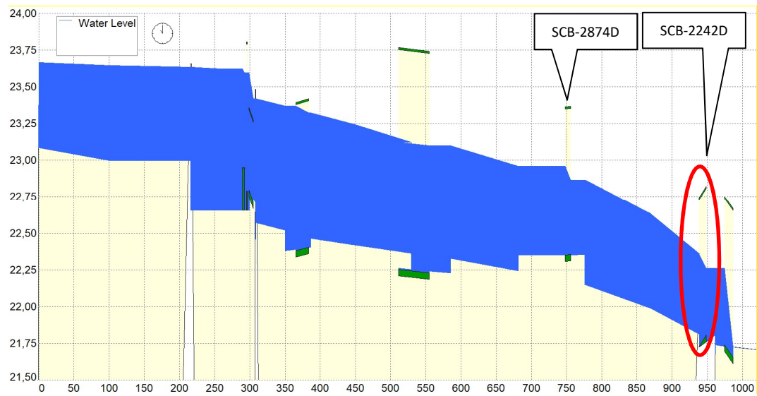
Figuur 4-1: Situatie Gansbeek vanaf waterberging tot duiker SCB-2247D - T50 winterbui situatie in huidige situatie. Ligging duiker SCB-2242D is niet correct gemodelleerd, duiker bevindt zich op de correcte manier in de stroomrichting.
