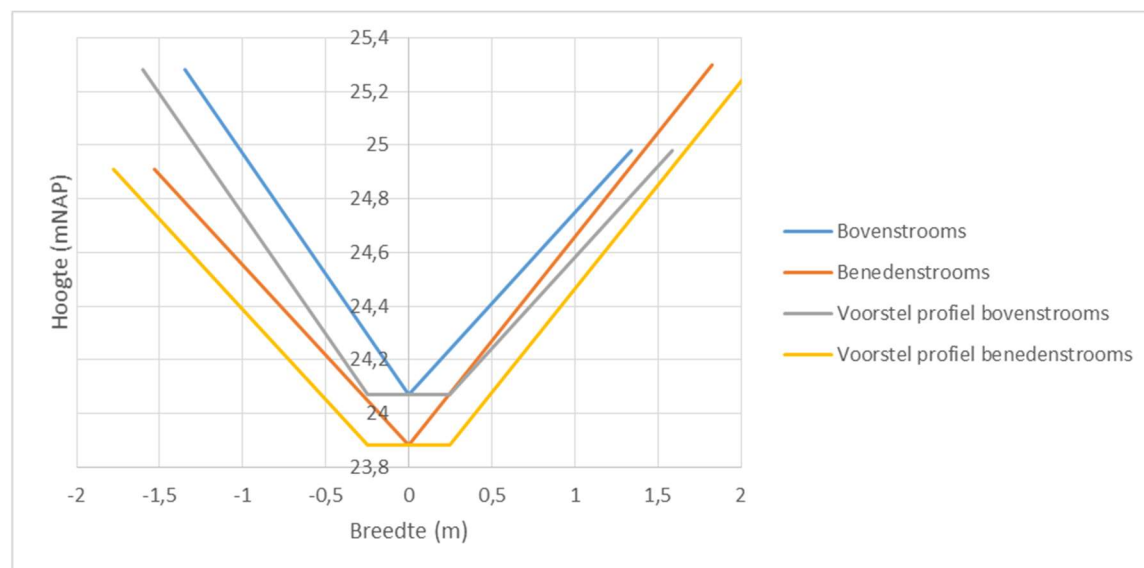
Figuur 2-11: Huidige profielen en voorgestelde profielen watergang Schelkensbeek tot Meerlebroek, bovenstrooms is profiel F, benedenstrooms is profiel G (zie bijlage 2)
