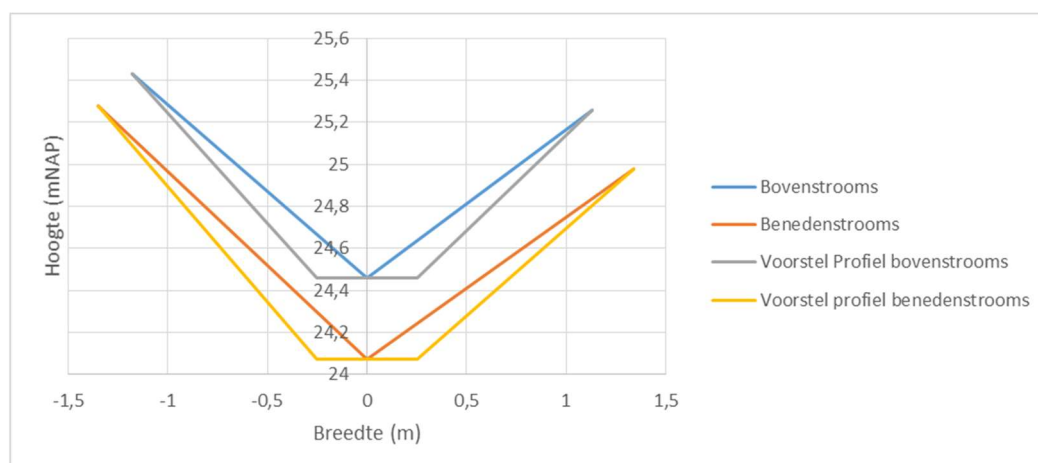
Figuur 2-9: Huidige profielen en voorgestelde profielen secundaire watergang Schelkensbeek, bovenstrooms is profiel E, benedenstrooms is profiel F (zie bijlage 2)
