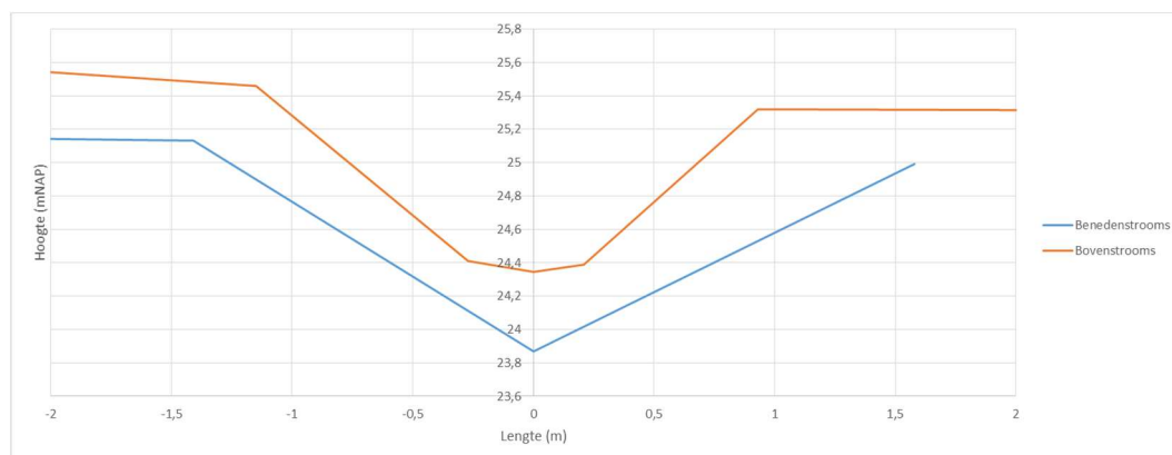
Figuur 2-7: Huidige profielen Meerlebroek, bovenstrooms is profiel C, benedenstrooms is profiel D (zie bijlage 2)
