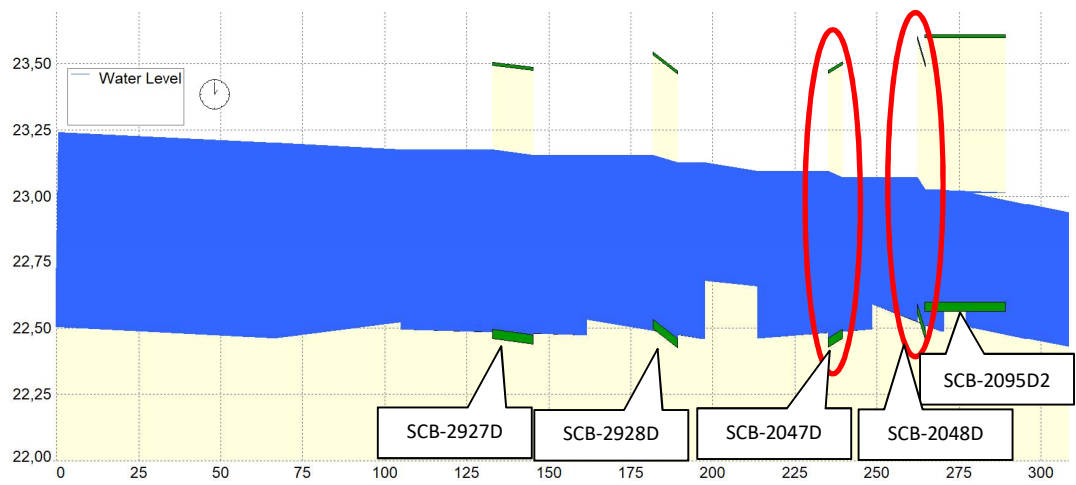
Figuur 3-3: Verloop bodemprofiel watergang Schelkensbeek, waarbij de duikers in de rode cirkels vervangen moeten worden – 0,5 MA.
