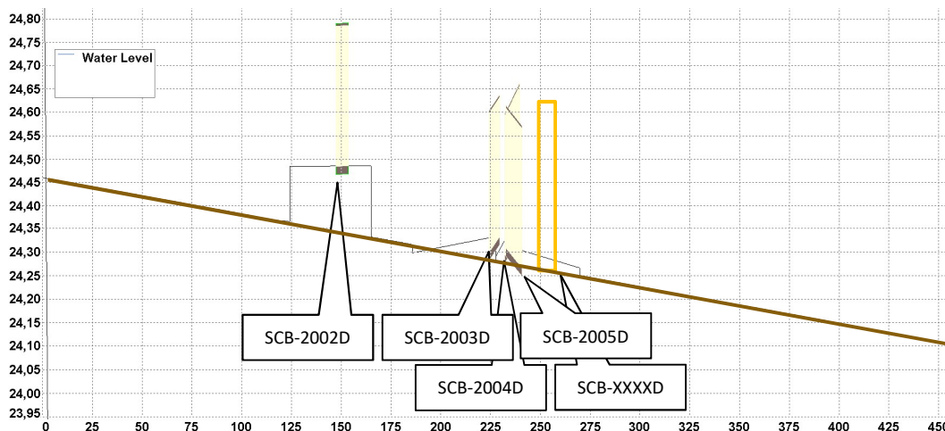
Figuur 2-8: Verloop bodemprofiel Secundaire watergang Schelkensbeek, waarbij alle duikers vervangen dienen te worden. Ook zijn er van één duiker geen gegevens bekend (oranje vierkant op 250 m).
