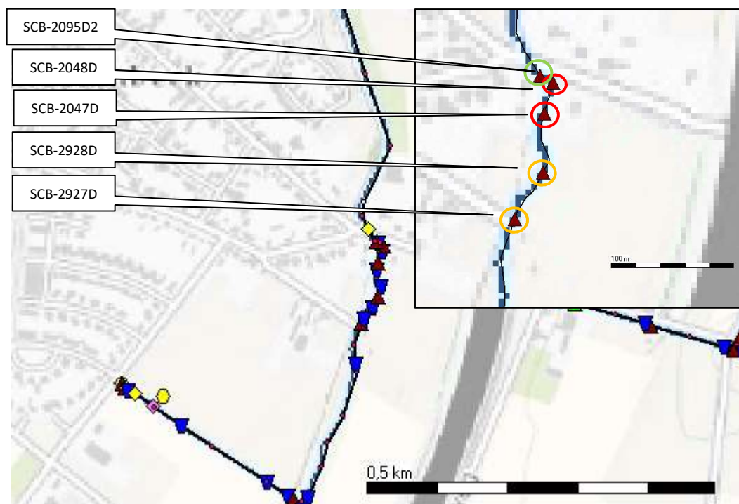
Figuur 3-2: Schematisatie situatie Schelkensbeek, met in rode cirkels de te verwijderen duikers, in oranje de duikers met dezelfde afmetingen en in groen de grootste duiker van de watergang.
