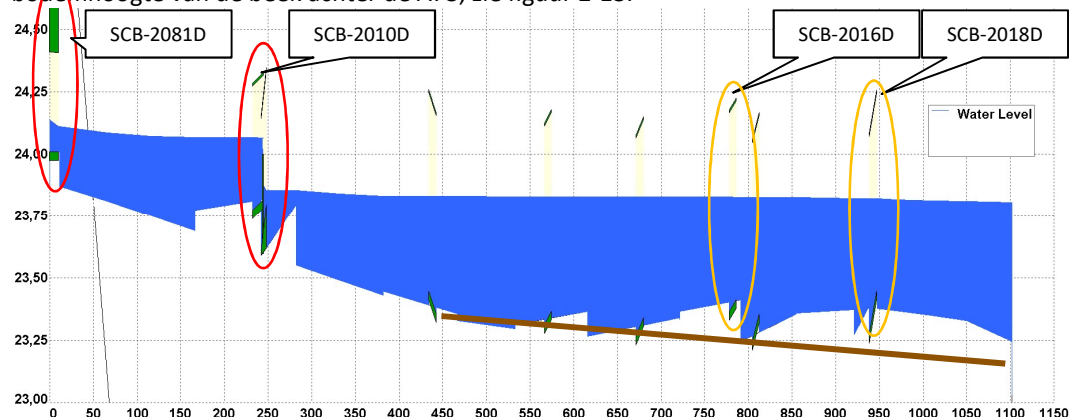
Figuur 2-12: Verloop bodemprofiel watergang Schelkensbeek, waarbij de duikers in de rode cirkels vervangen moeten worden – 0,5 MA
