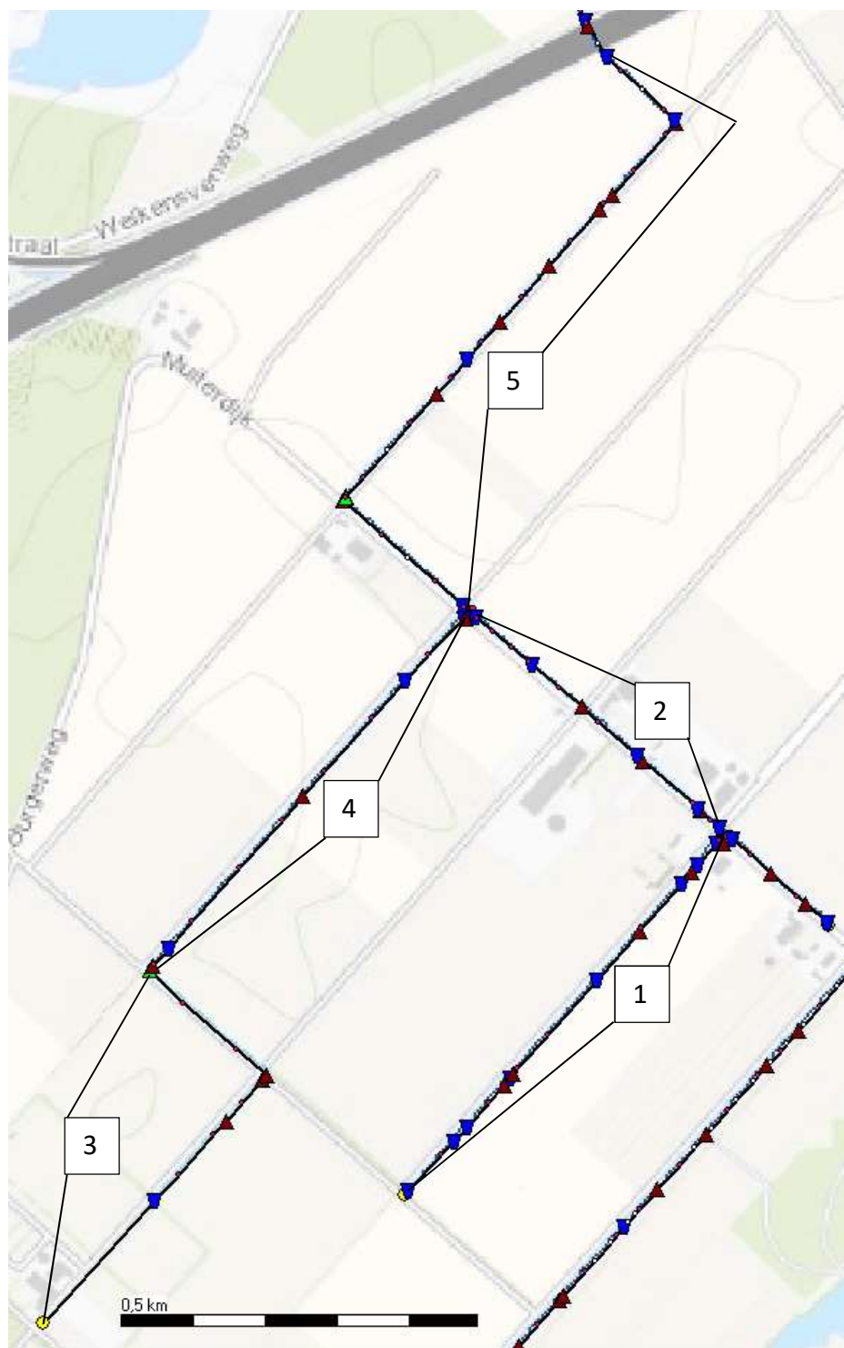
Figuur 2-3 Situatie bovenstrooms Schelkensbeek – De hydrologische situatie is per watergang (1 t/m 5) onderzocht en de watergang gedimensioneerd.
