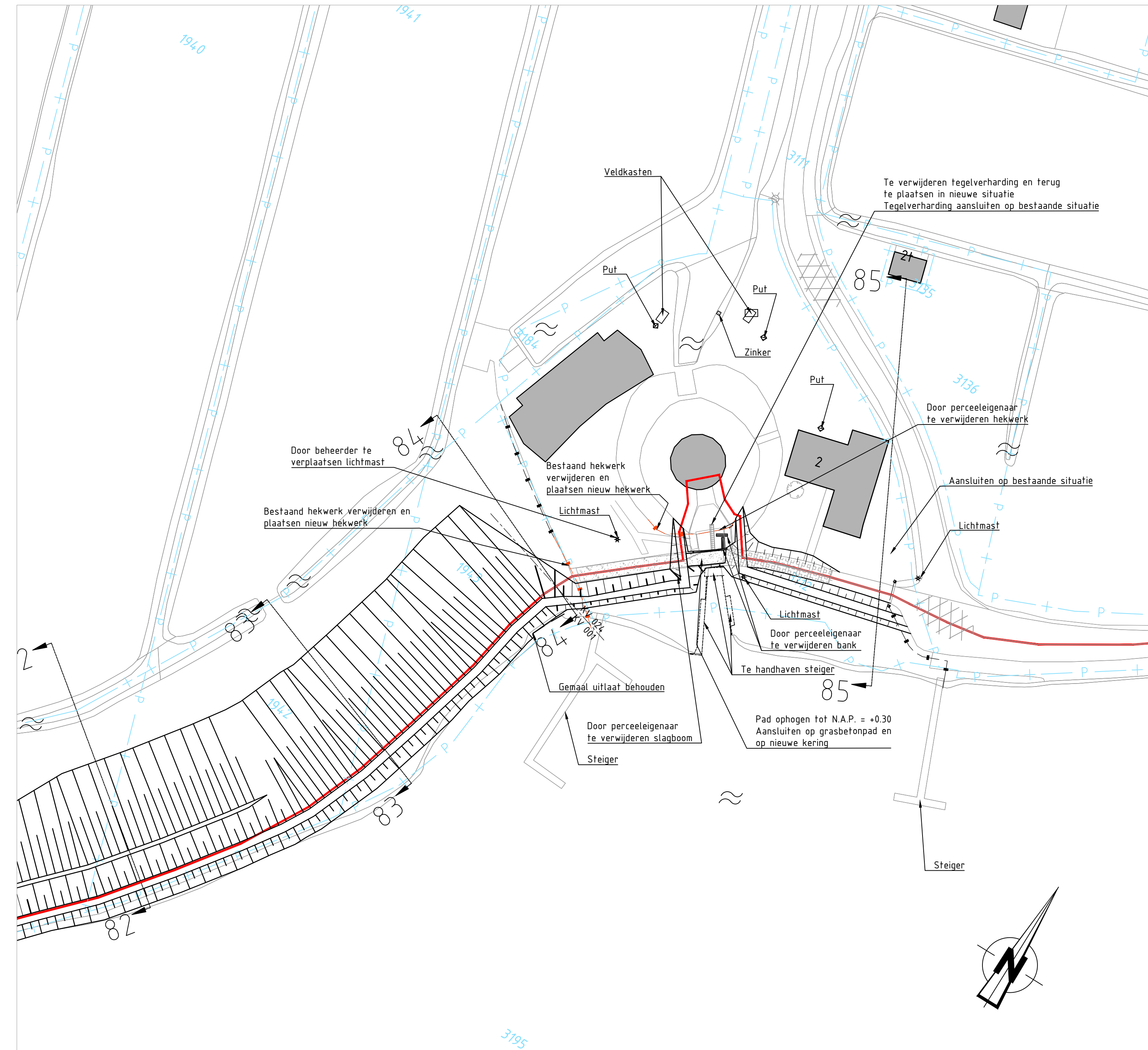
Bovenaanzicht Veenderpolder DV 05 Schaal 1:500
