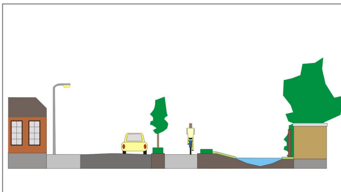
Profiel middengedeelte van het Keern
