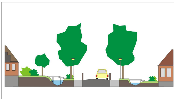
Profiel Dorpsstraat West
