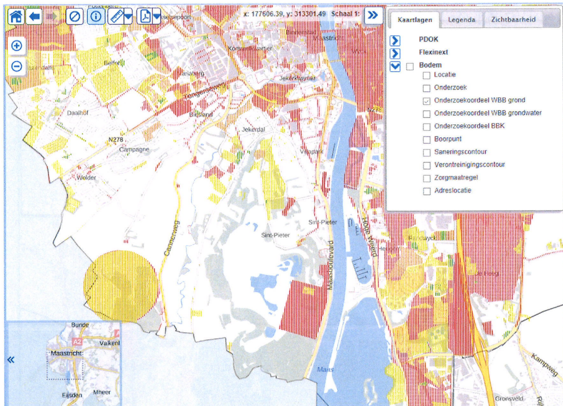
Figuur 4.6 Grondverontreinigingen aangetroffen in tijdens bodemonderzoeken in de omgeving van de ENCI-groeve
