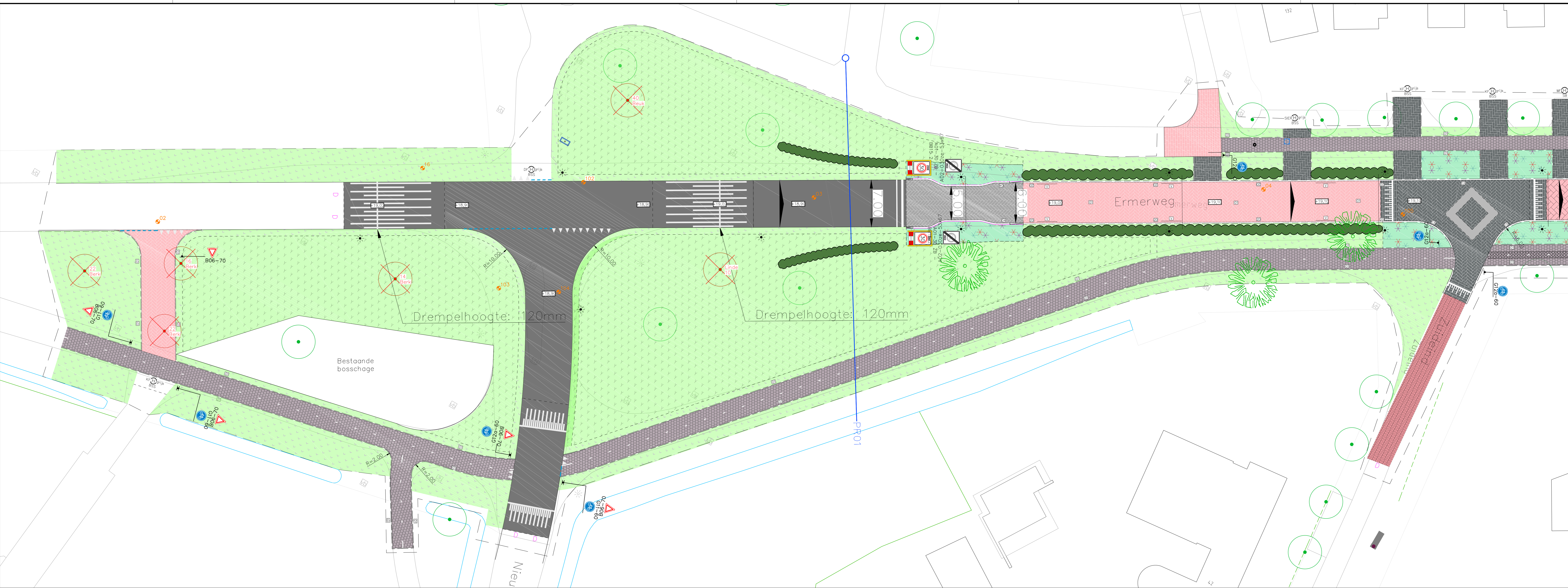
SITUATIE 001 SCHAAL 1:200
