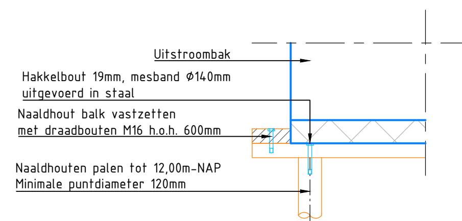
Detail 1: Aansluiting houten palen op badding SCHAAL 1:20
