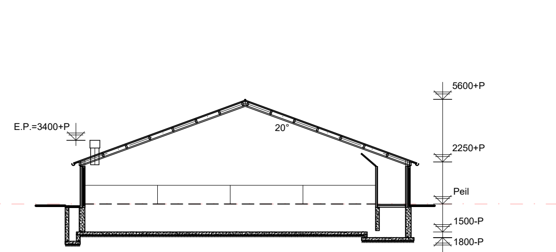
DOORSNEDE A-A GEBOUWNR 1
