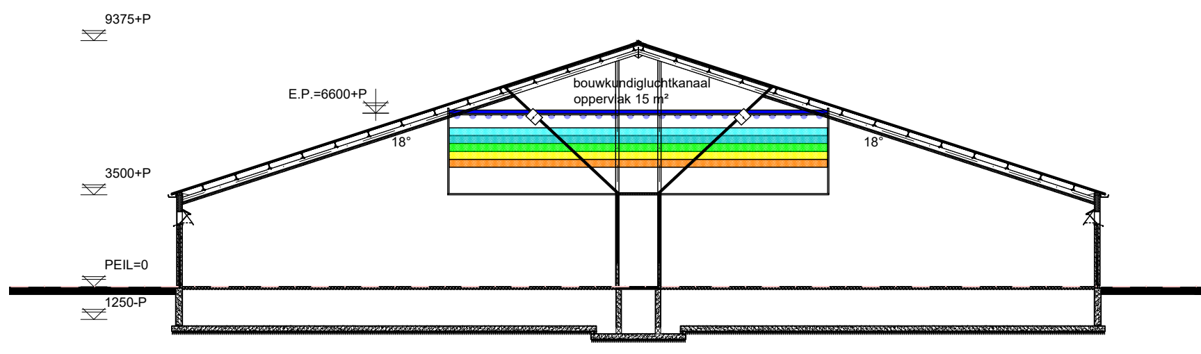
DOORSNEDE B-B GEBOUWNR 2
