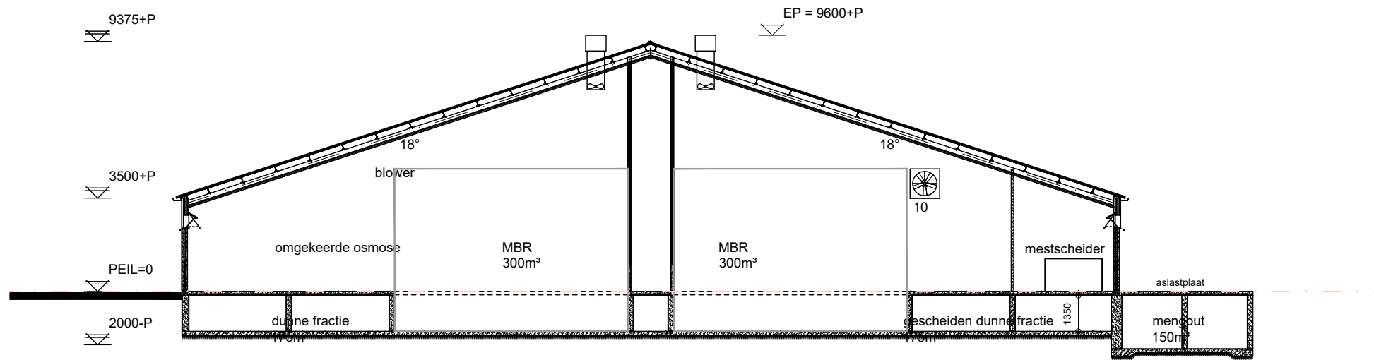
DOORSNEDE B'-B' GEBOUWNR 2
