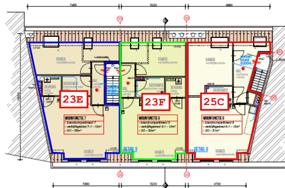
DERDE VERDIEPING NIEUWE SITUATIE
