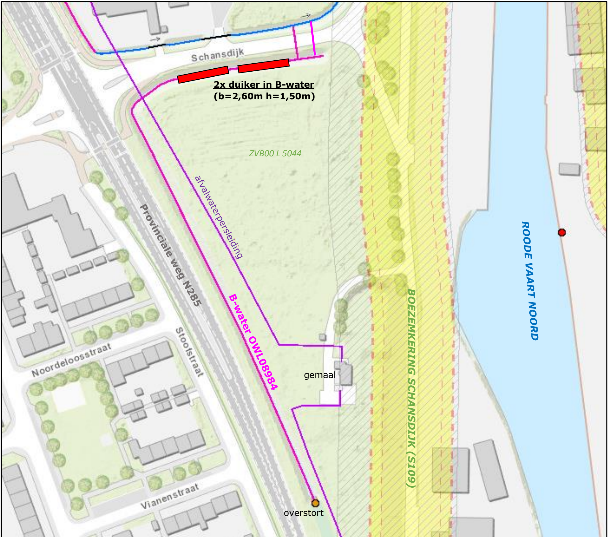
341948-A Topografische situatie
