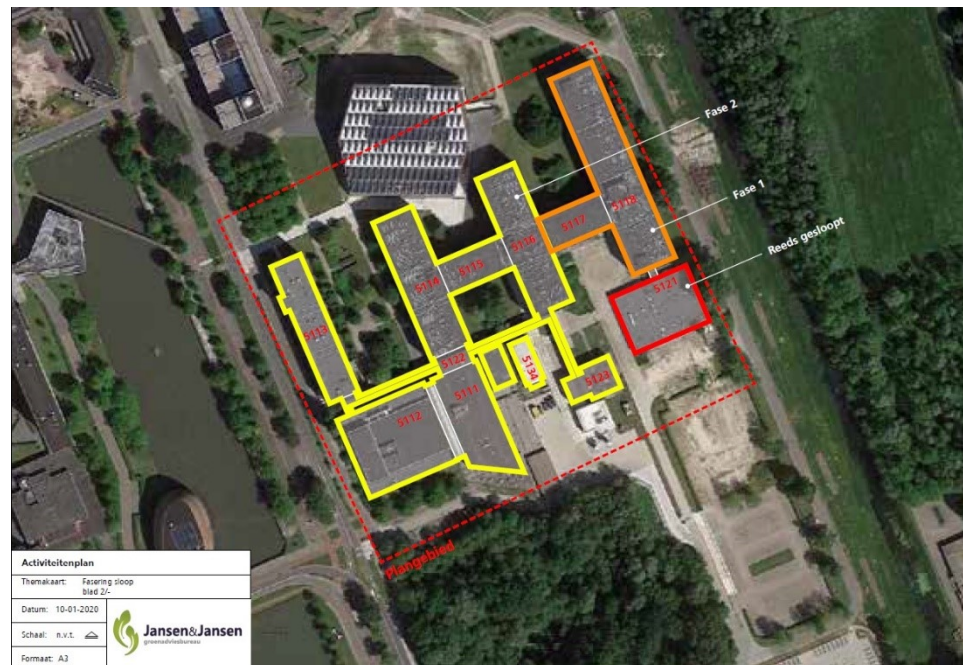
Figuur 2. Faseringsloop FWN-gebouw (oranje: fase 1, geel: fase 2, rood: reeds gesloopt). Bron: Activiteitenplan Jansen & Jansen, 16 september 2020.
