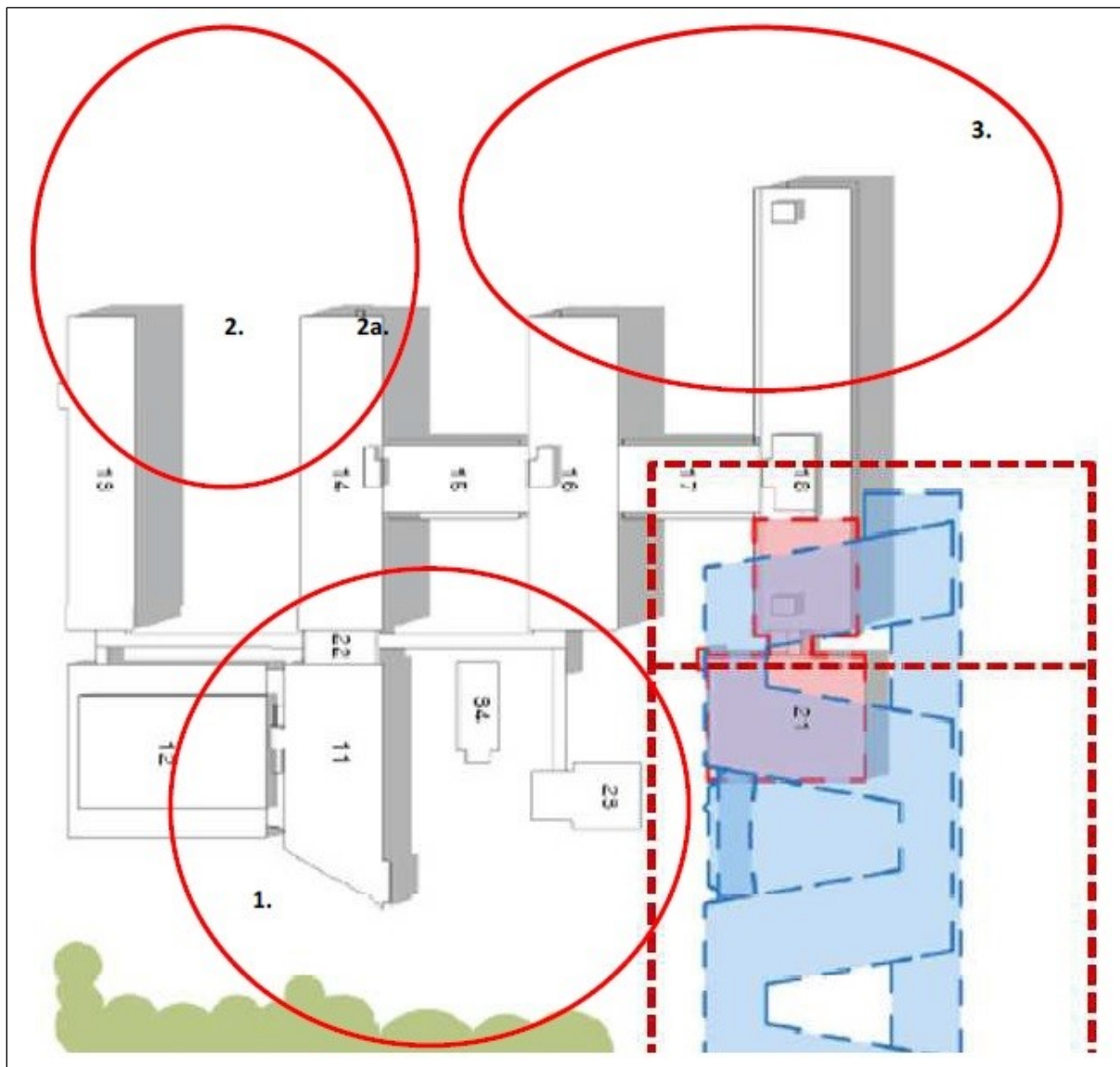
Figuur 3. Overzicht baltterritoria Gewone dwergvleermuis rond het FWN-gebouw (nummers 1 t/m 3). Op locatie 2a is in de voorzomer kort een zwermende Gewone dwergvleermuis waargenomen (betreft een mogelijke zomerverblijfplaats).
