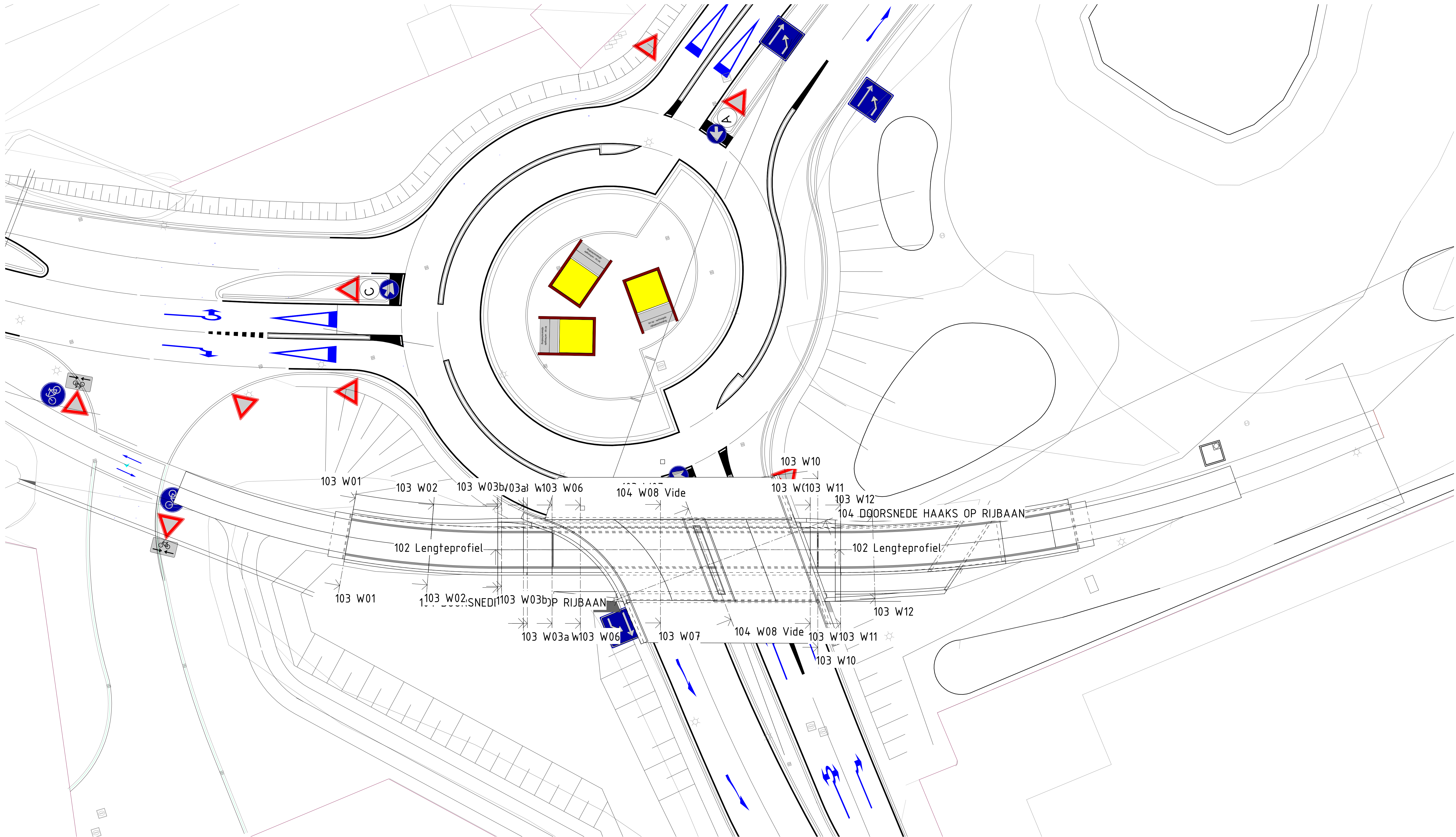
101 Situatie SCHAAL: 1 : 200
