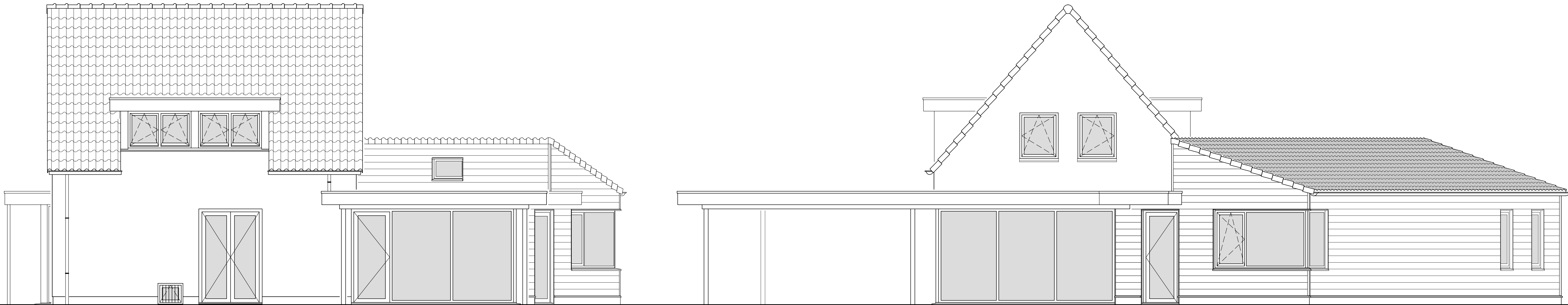
≈ Zuid-Oostgevel ≈
