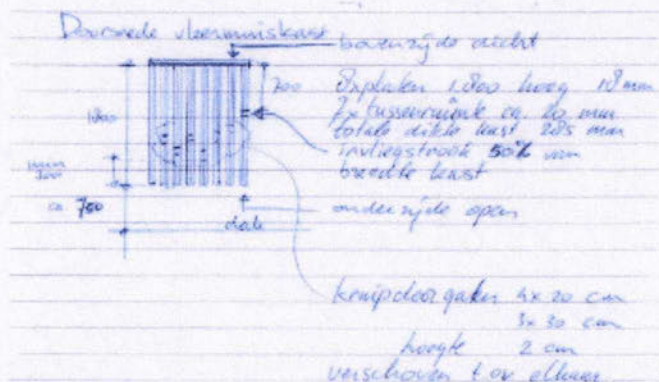
Figuur 28. Technische schets van de winterverblijfsvoorziening in het provinciehuis in Zwolle; voorziening Duivenwal wordt op dezelfde wijze vormgegeven.
