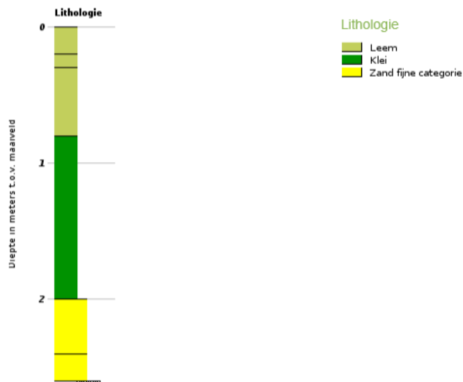
Figuur 8: Boorprofiel ter hoogte van de Waterstraat
