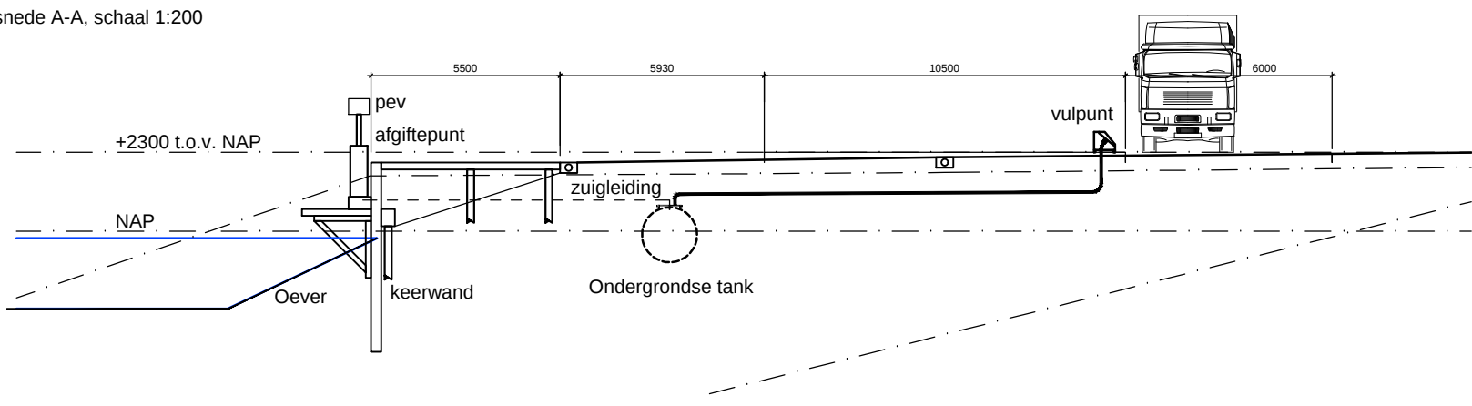
Doorsnede A-A, schaal 1:200
