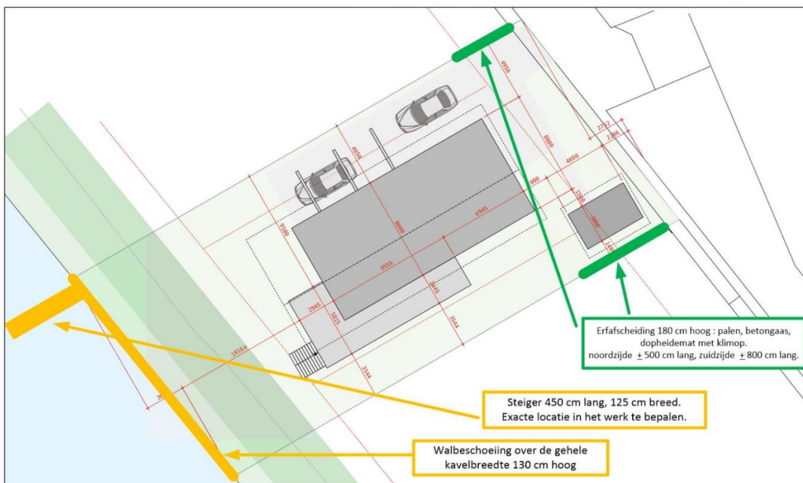
Bovenaanzicht
