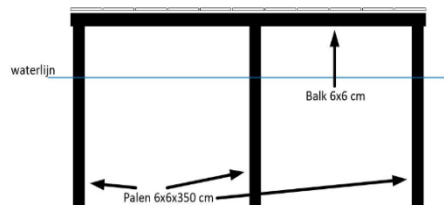
Zij-aanzicht
