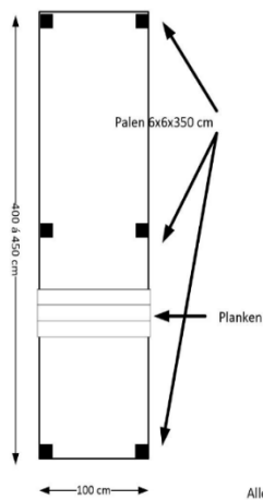
Bovenaanzicht
