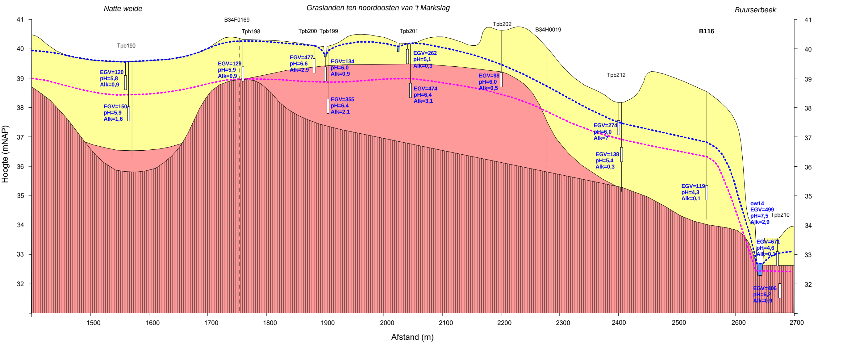
Figuur 4.1a Ecohydrologisch dwarsprofiel A-A' (voor legenda: zie figuur 4.1d)
