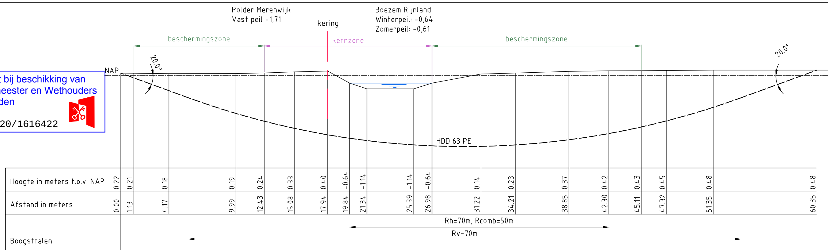
Doorsnede A-A, schaal 1:200
