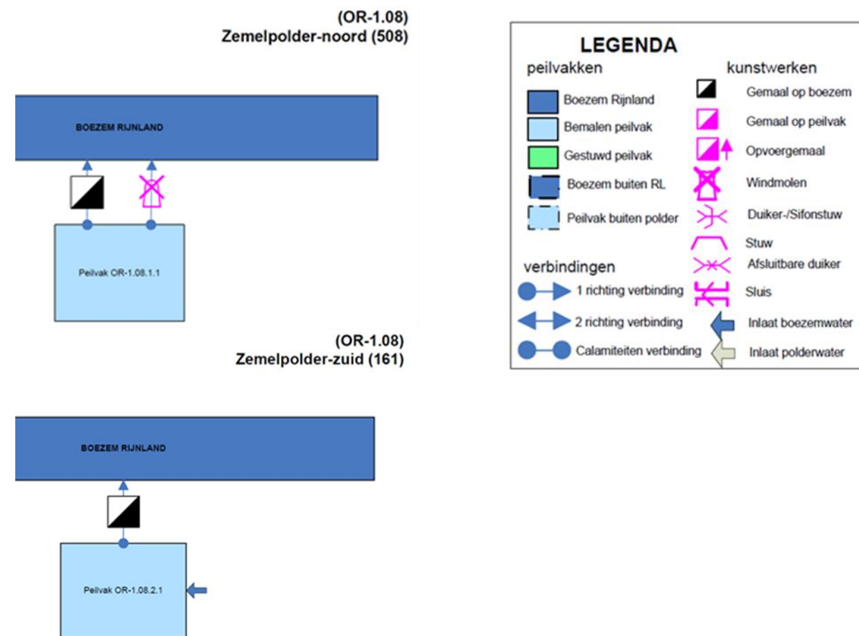
Figuur 3-8 Theoretisch aan- en afvoerschema peilvakken Zemelpolder
