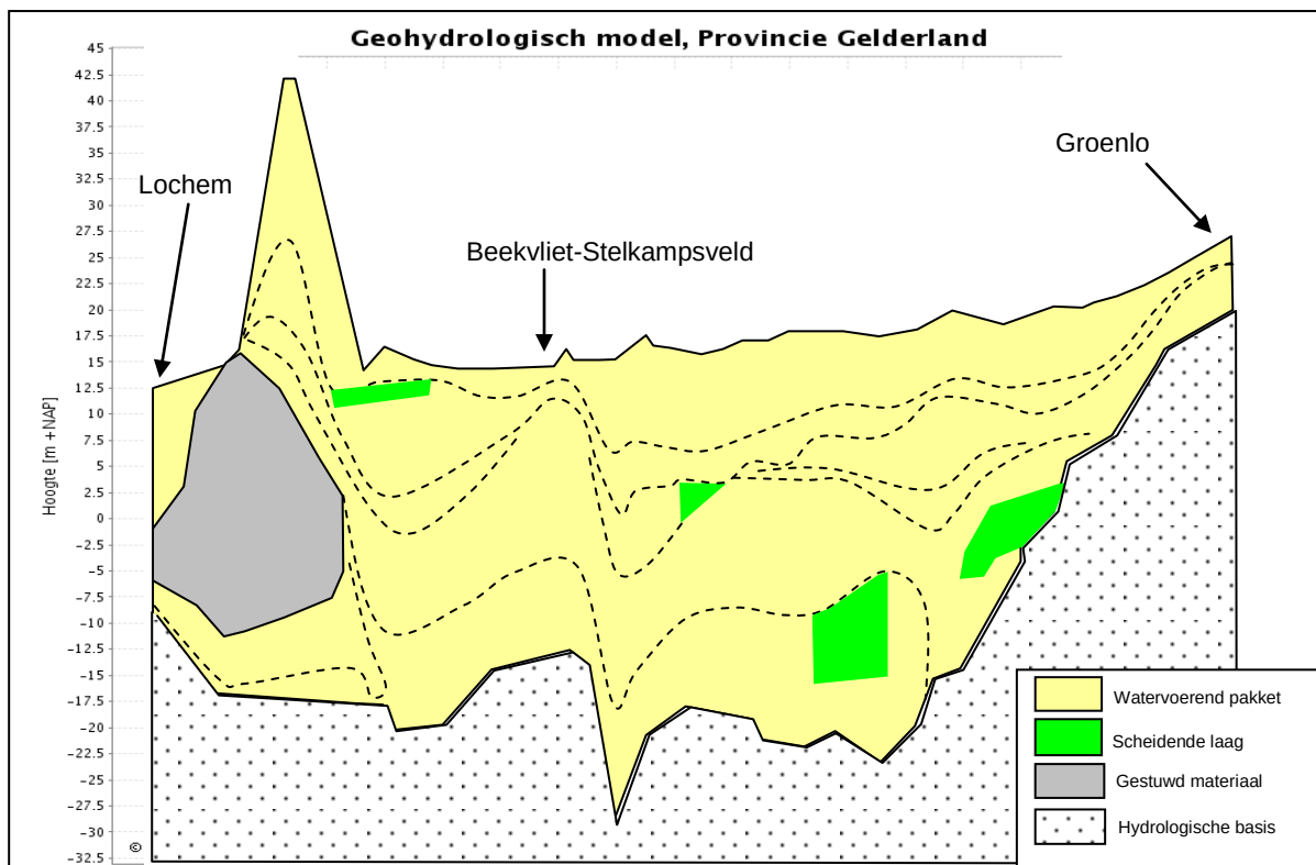
Figuur 3 Geohydrologische dwarsdoorsnede van Groenlo naar Lochem (bron: REGIS II, TNO)
