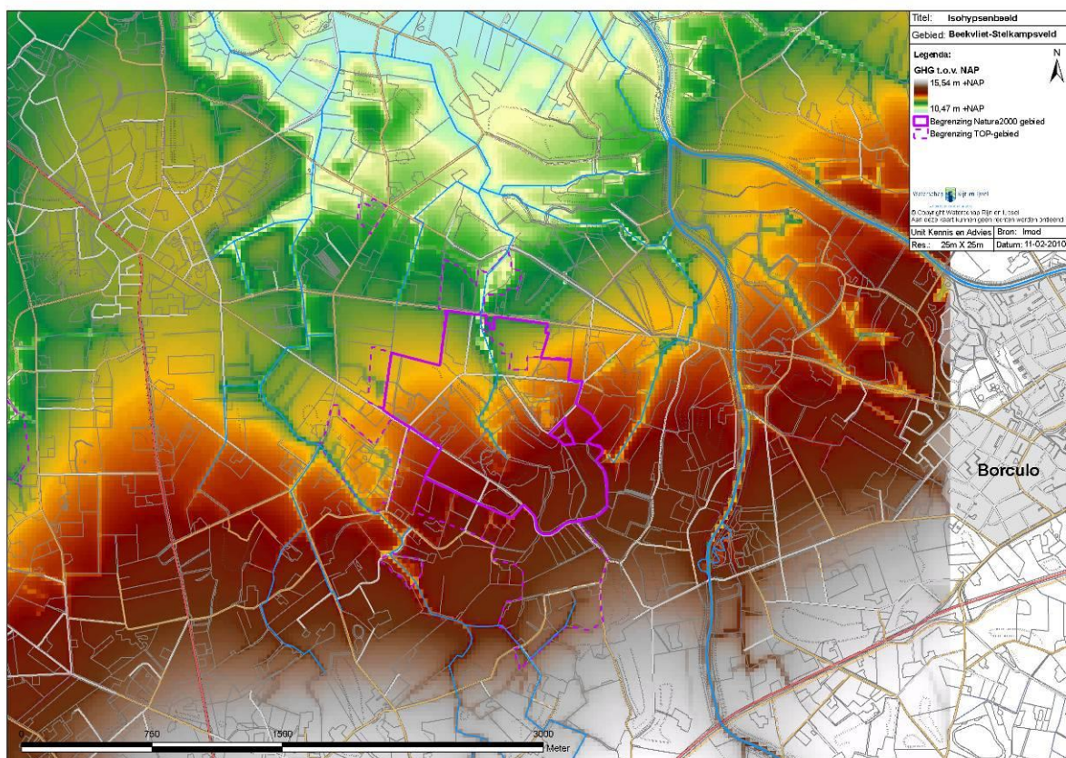
Figuur 4 Isohypsensbeeld rondom Beekvluit-Stelkampsveld: water stroomt dwars op de isohypsen, van hoge naar lage stijghoogte
