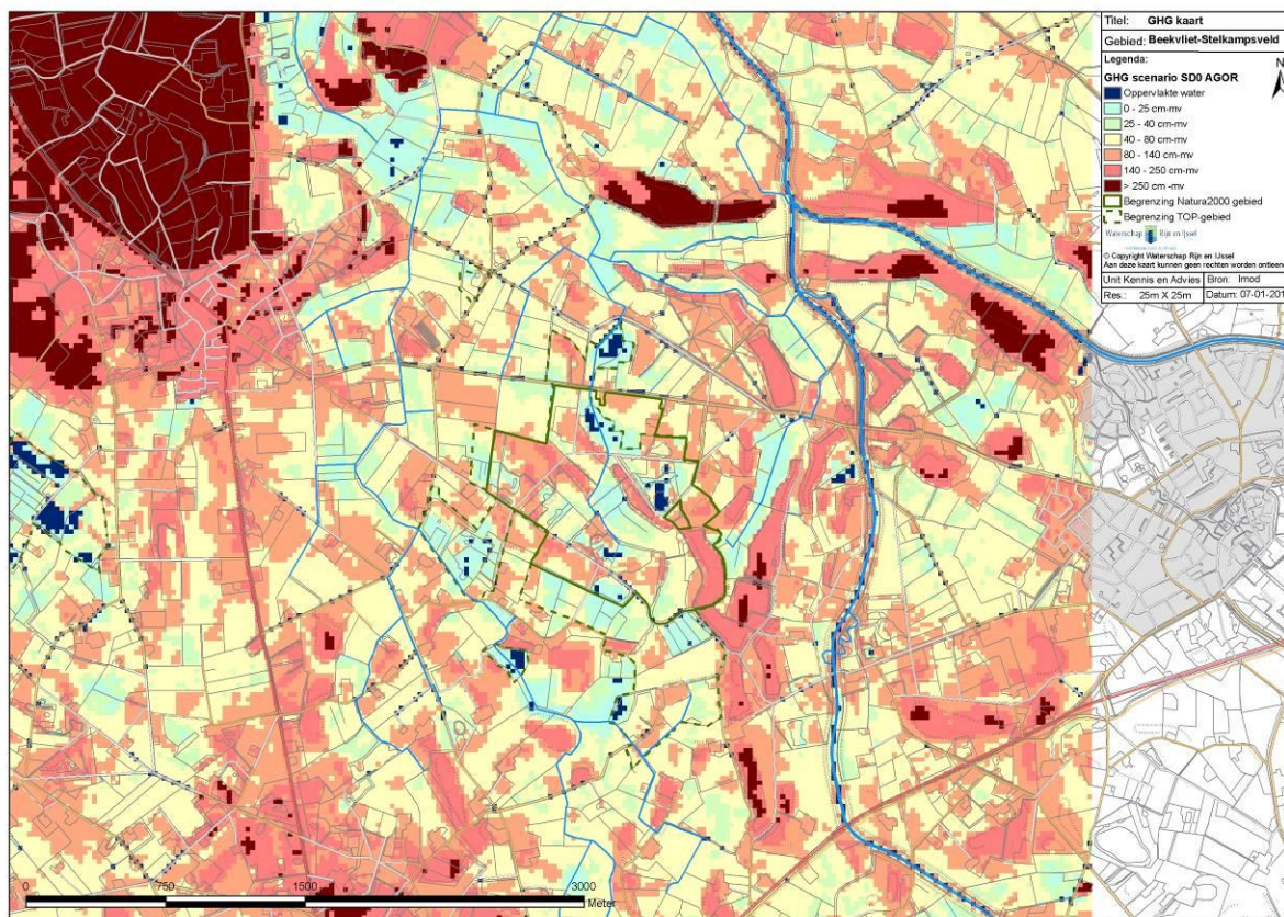
Figuur 6 Beeld van de GHG (gemiddeld hoogste grondwaterstand) in het gebied Beekvliet-Stelkampsveld zoals berekend met Amigo
