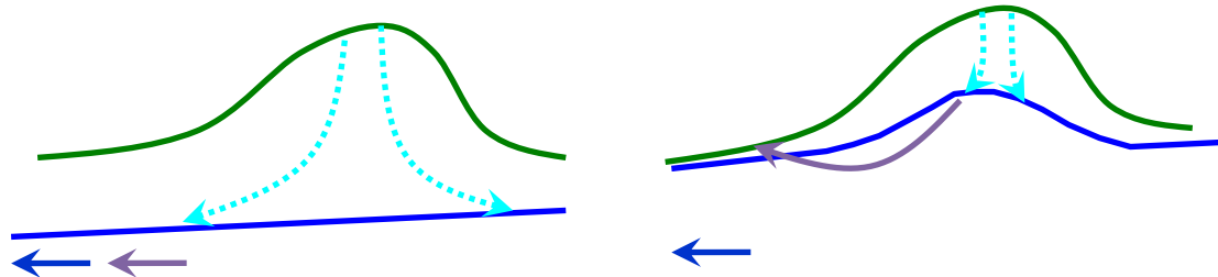
Figuur 5 Superpositie van tijdelijke, lokale systeemjes op het regionaal grondwatersysteem neerslag infiltreert (lichtblauwe stippels) en stroomt verder (paars) als regionaal grondwater (links) of kwelwater in nabijgelegen laagte(rechts) donkerblauw: grondwaterniveau en stromingsrichting regionaal grondwater, paars: stromingsrichting recent geïnfiltreerd water, groen: maaiveld
