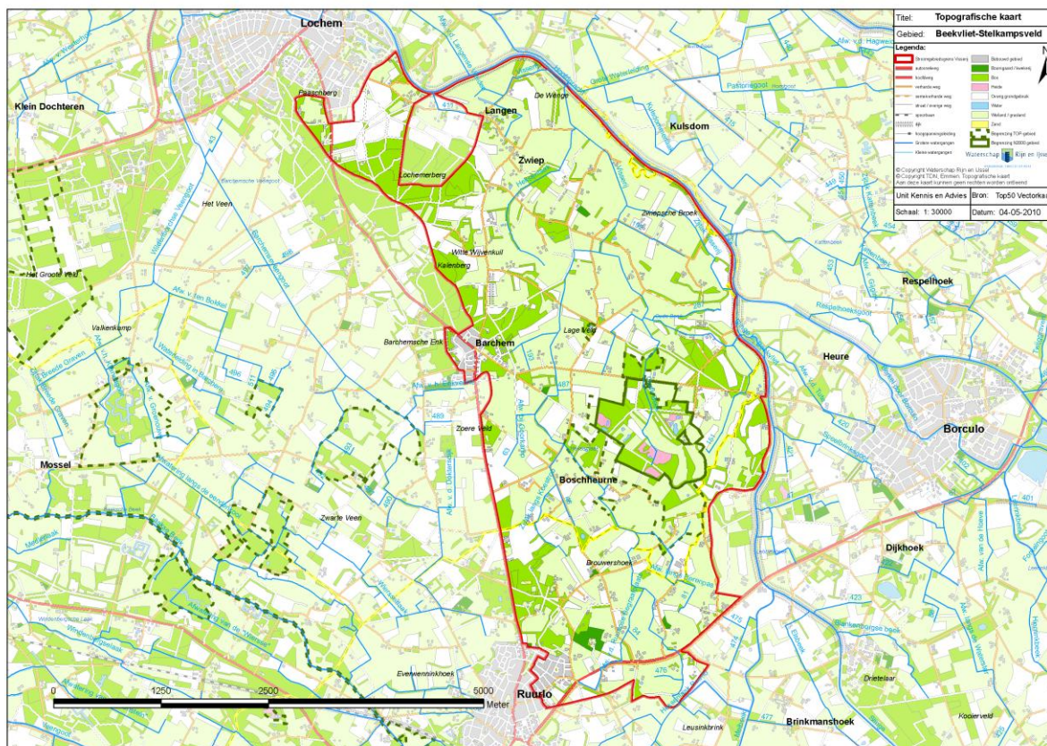
Figuur 1 Ligging gebied Beekvliet-Stelkampsveld tussen Borculo en Lochem, in het stroomgebied van de Visserij
