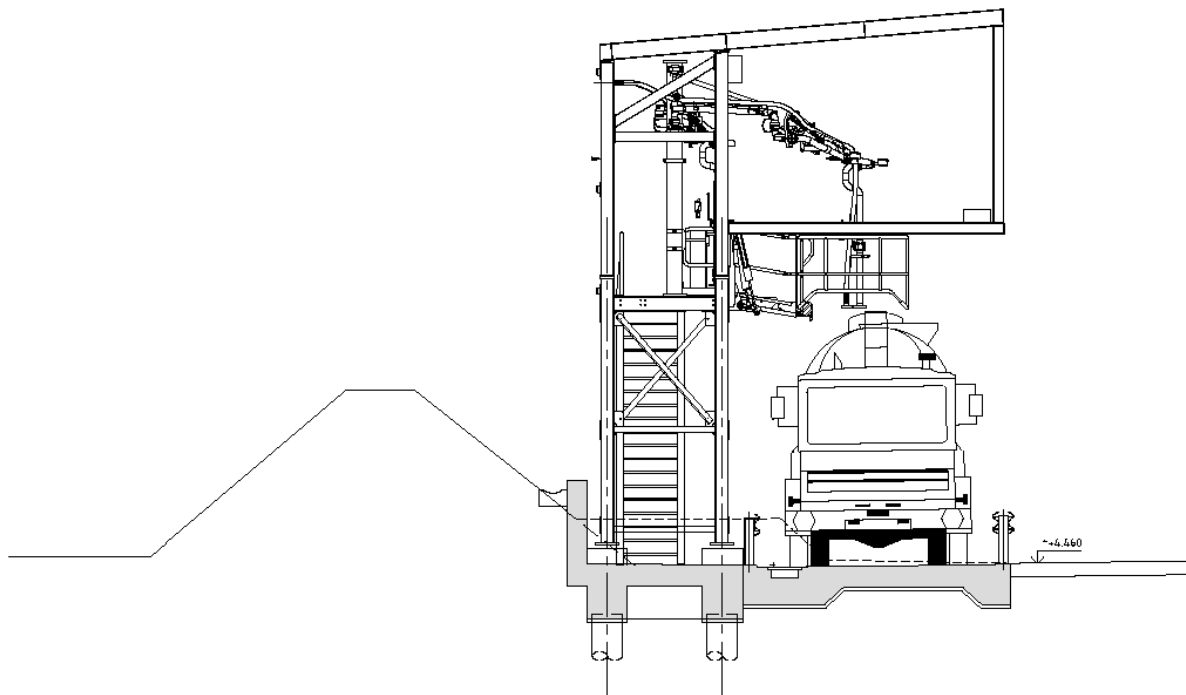
figuur 4: Constructie tarverladingsstation
