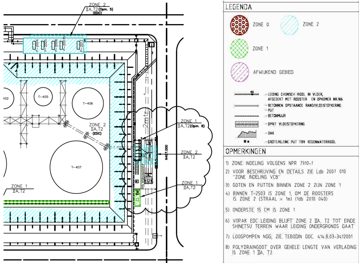
figuur 3 deel van de zoneringsstekening t.h.v. de nieuwe tarverladingsplaats
