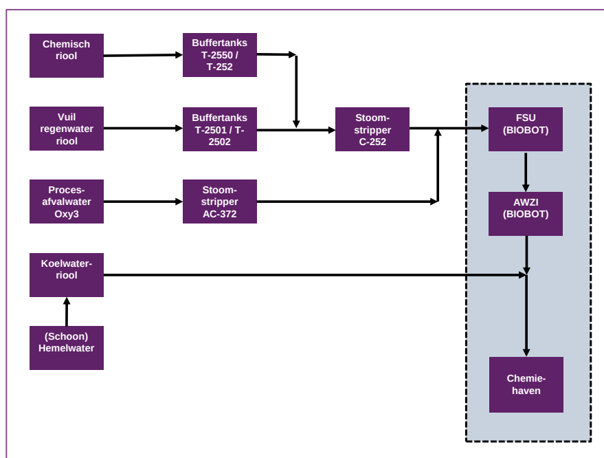
Figuur 2.1 Schematische weergave van het rioolstelsel
