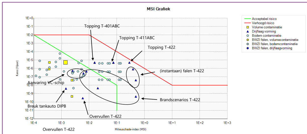
Figuur 5.3b Presentatie van installatie onderdelen met een risico op vorming van een drijfslag
