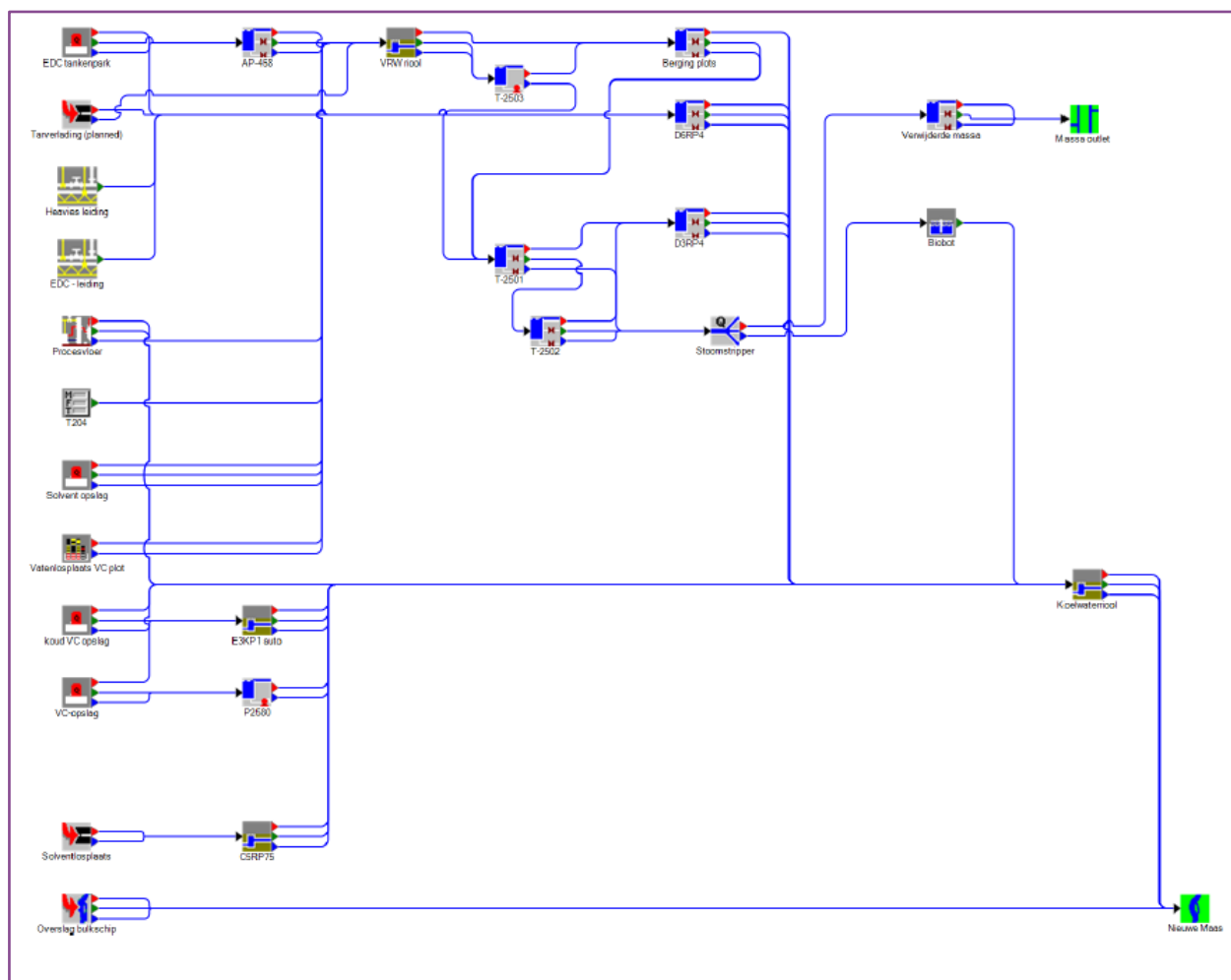
Figuur 5.1 Lozingspaden Proteus III model
