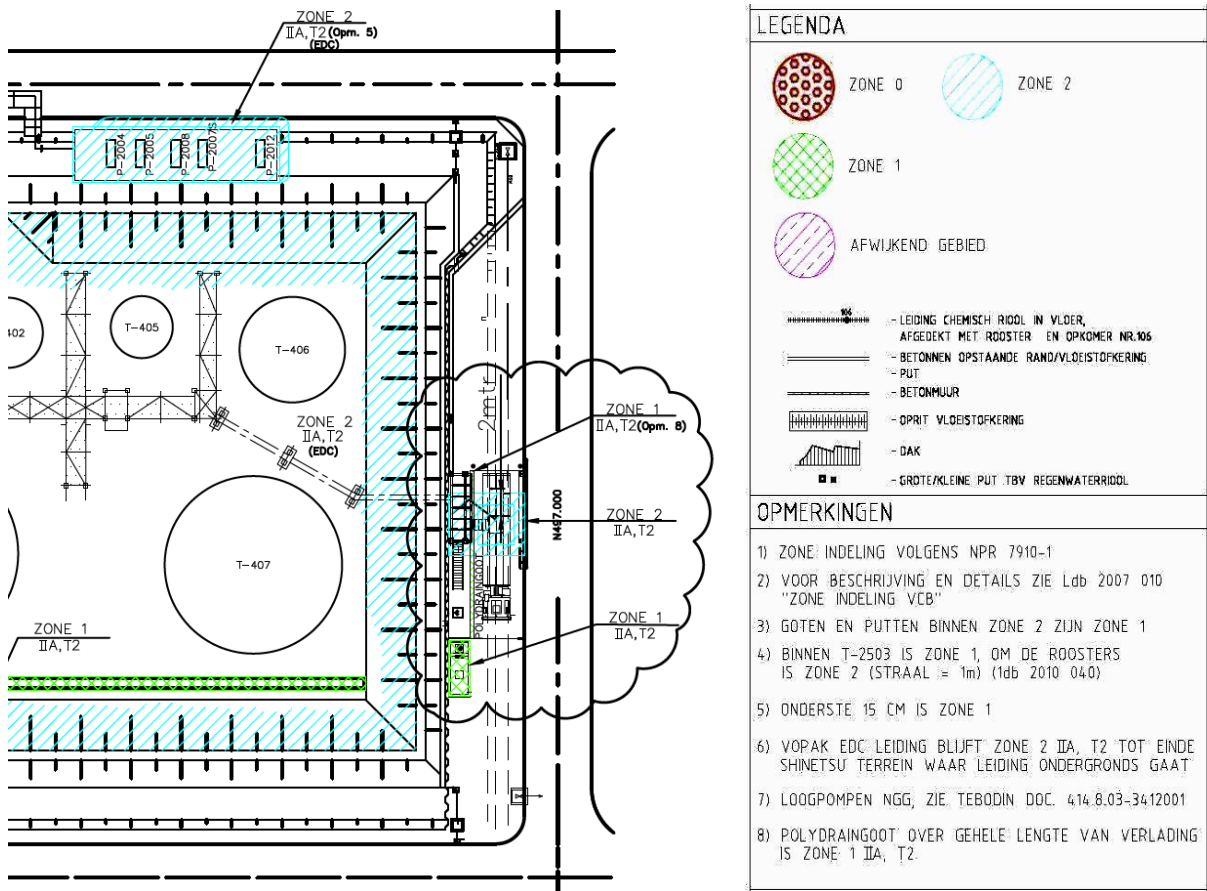
figuur 3 deel van de zoneringstekening t.h.v. de nieuwe tarverladingsplaats
