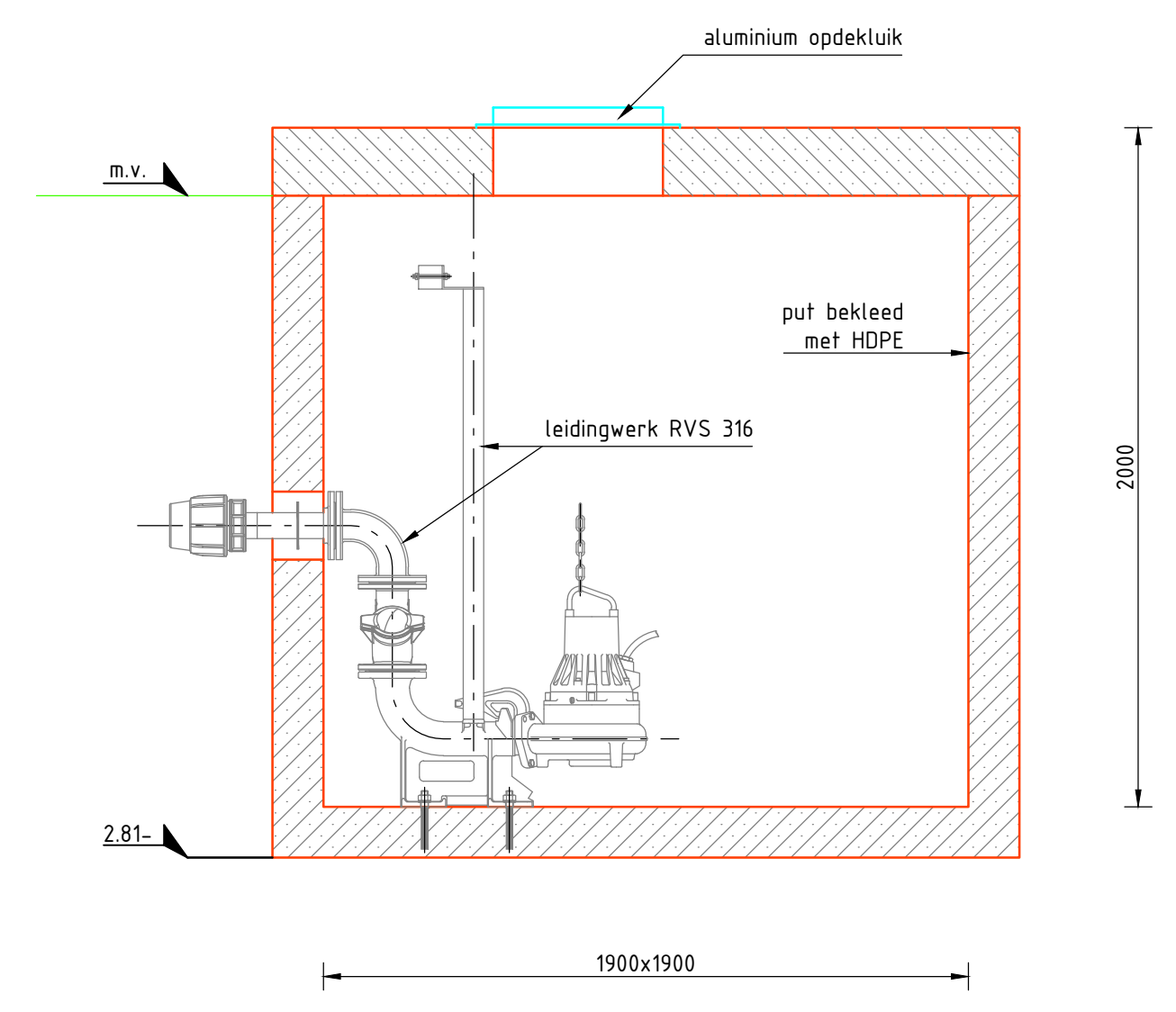
DETAIL RIOOLGEMAAL
