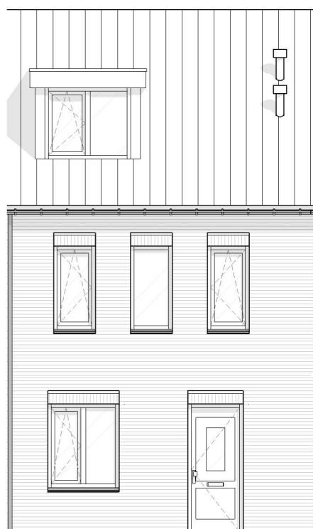
Gevel aanzicht
