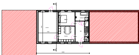
BEGANE GROND
