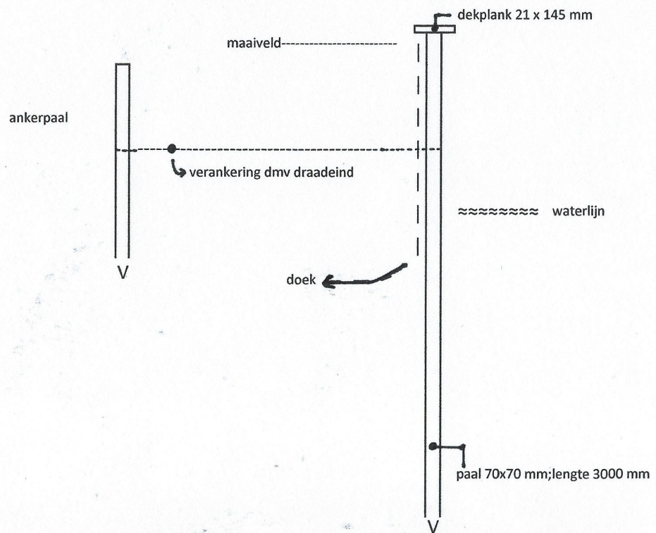
Zijaanzicht schoeiing
