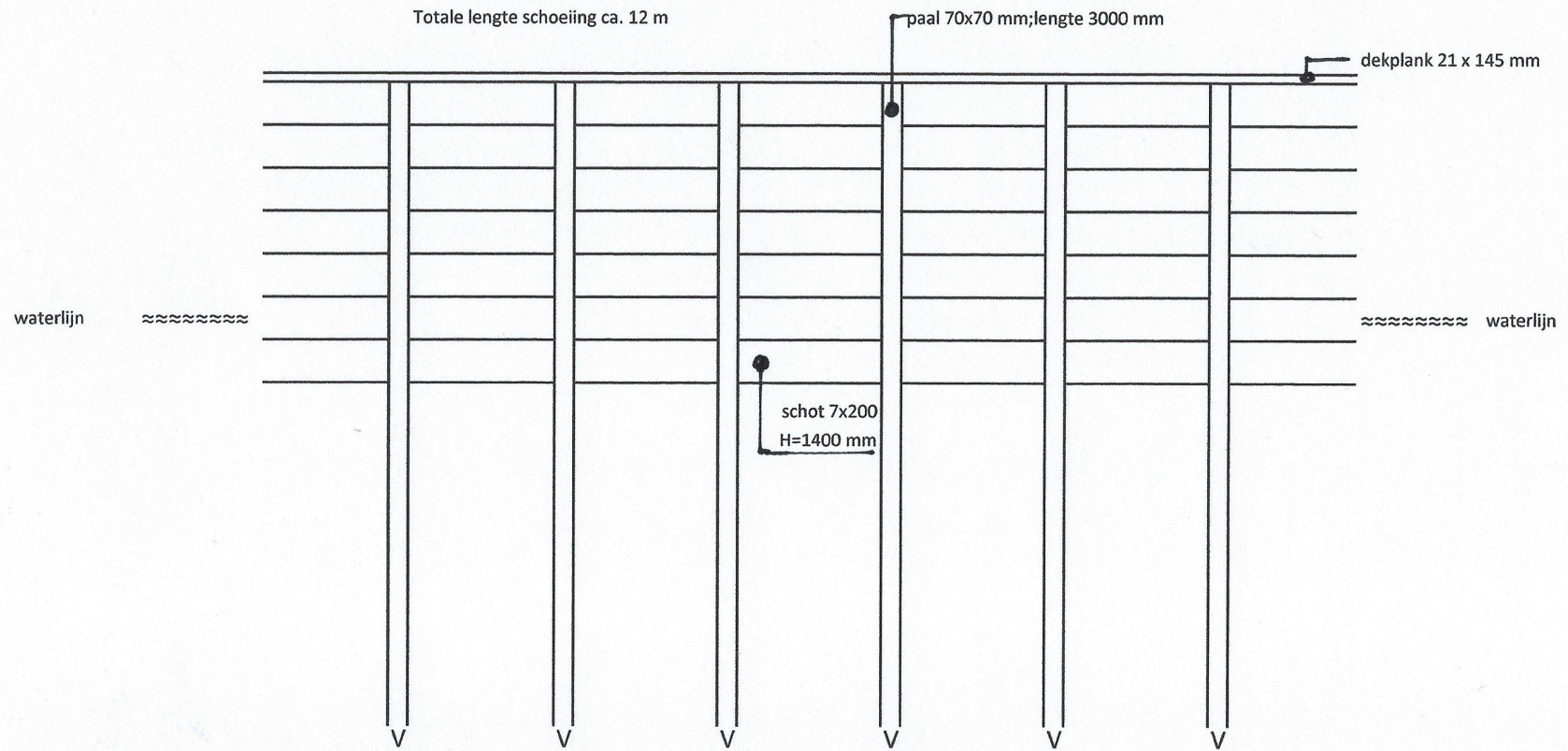
Vooraanzicht schoeiing
