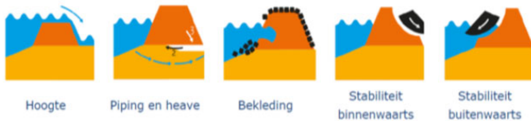
Figuur 0.1 Werking van de verschillende faalmechanismen
