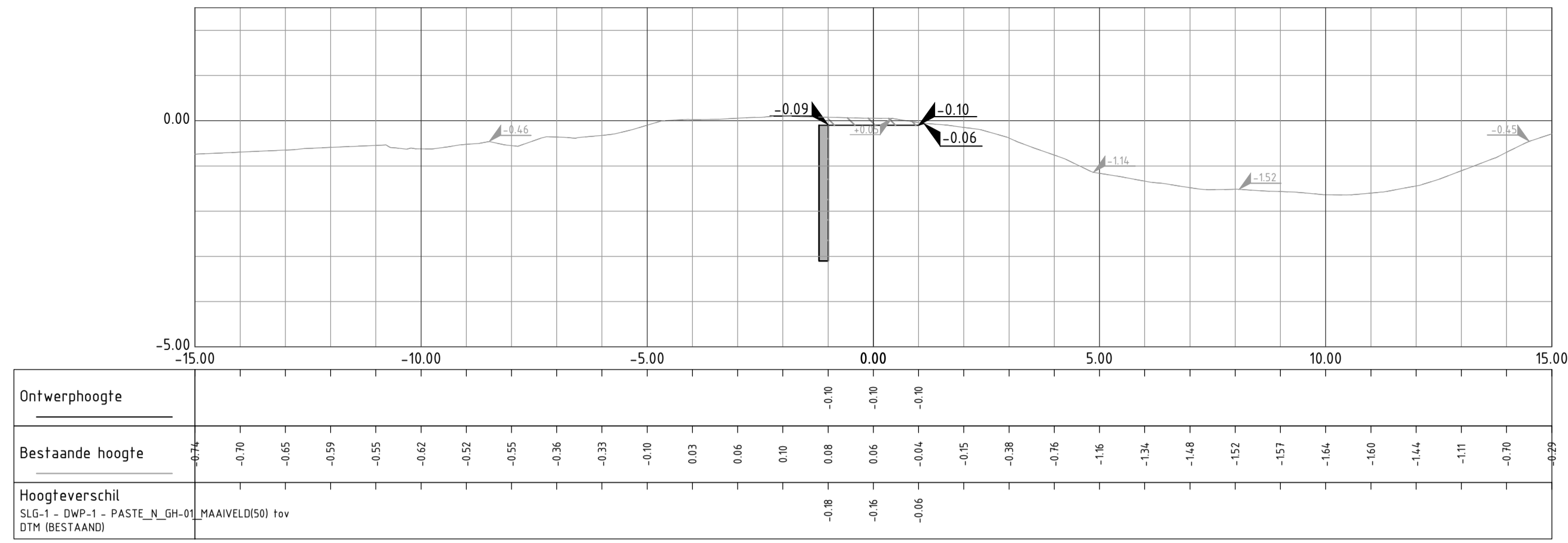
DWP-1 Schaal 1:100
