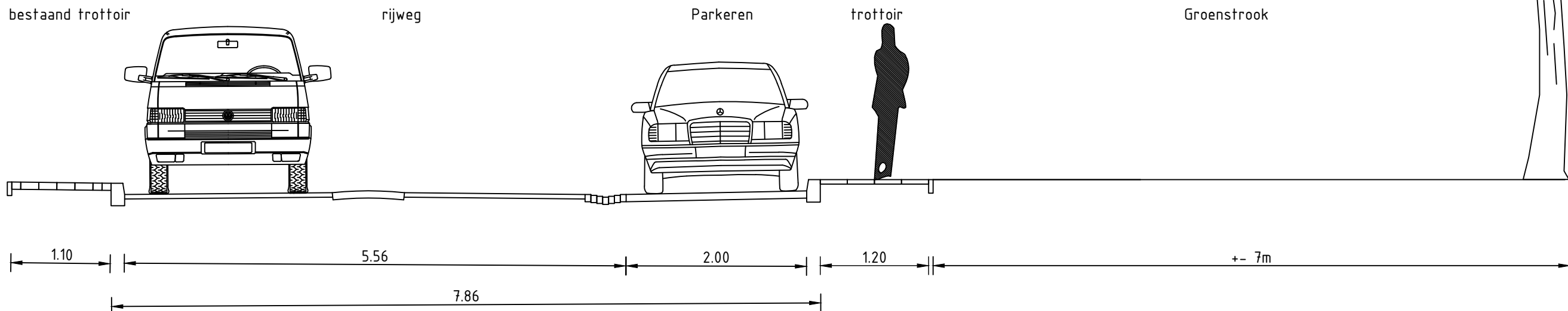
Doorsnede B-B SCHAAL 1 : 50
