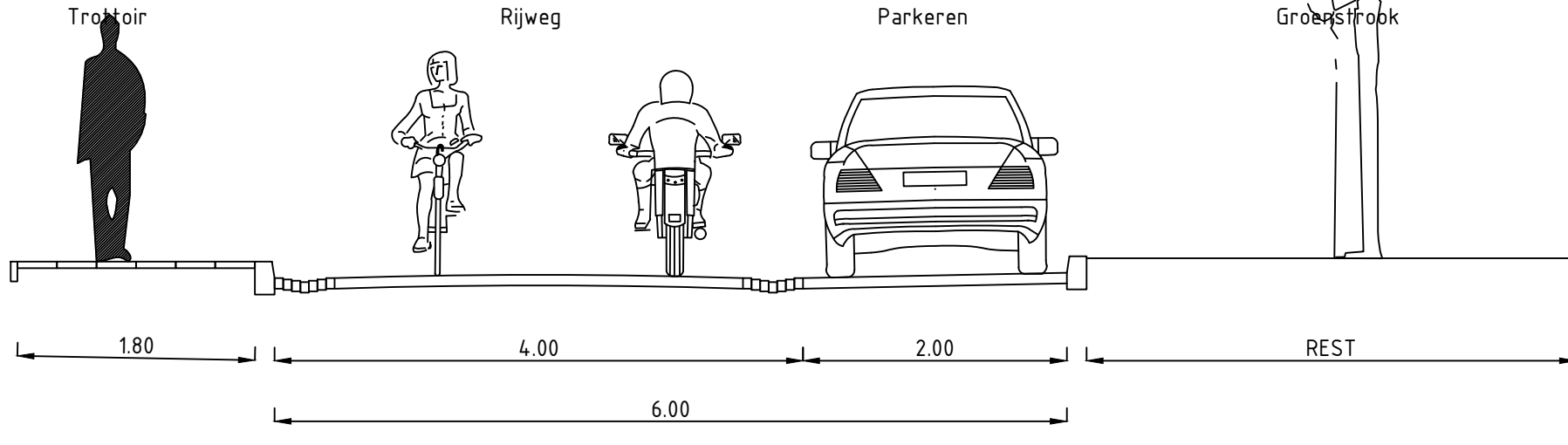
Doorsnede C-C SCHAAL 1 : 50
