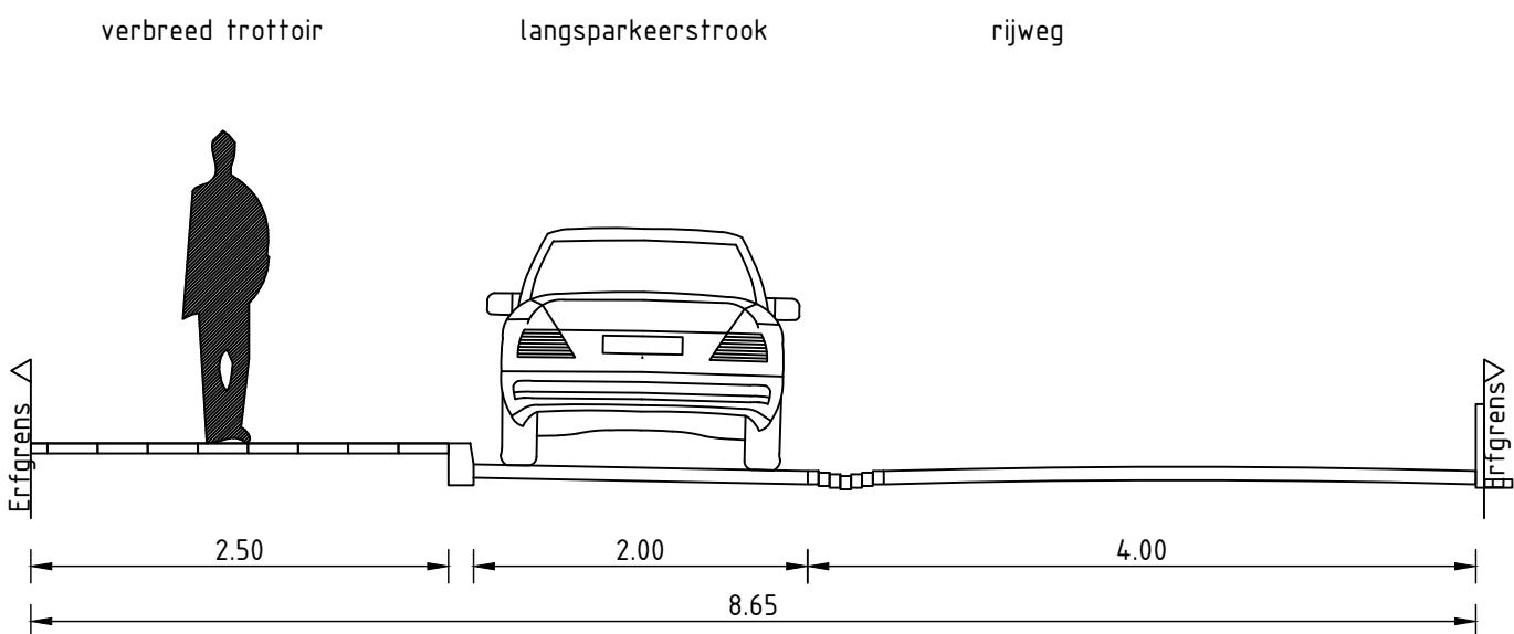
Doorsnede D-D SCHAAL 1 : 50
