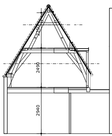
doorsnede
