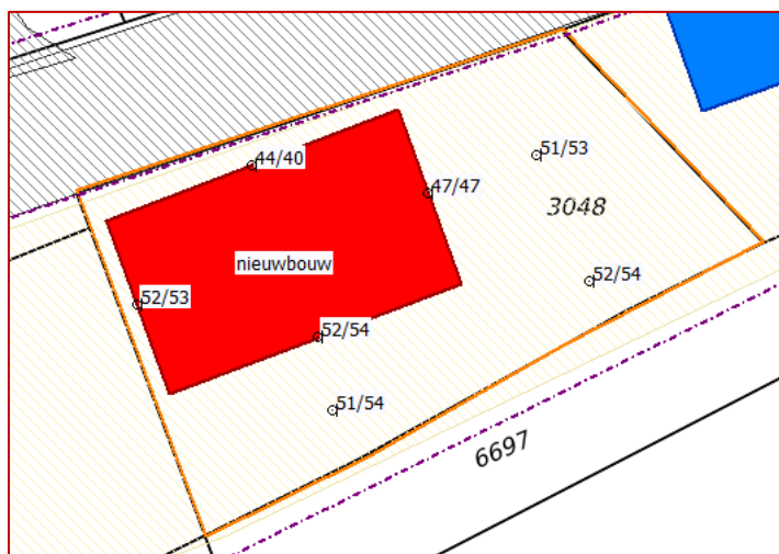
Figuur 5.2: Rekenresultaten vanwege spoorweglawaai inclusief buitenruimten
