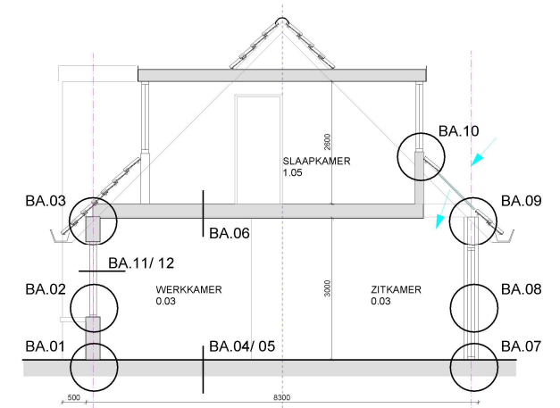
Overzicht details doorsnede
