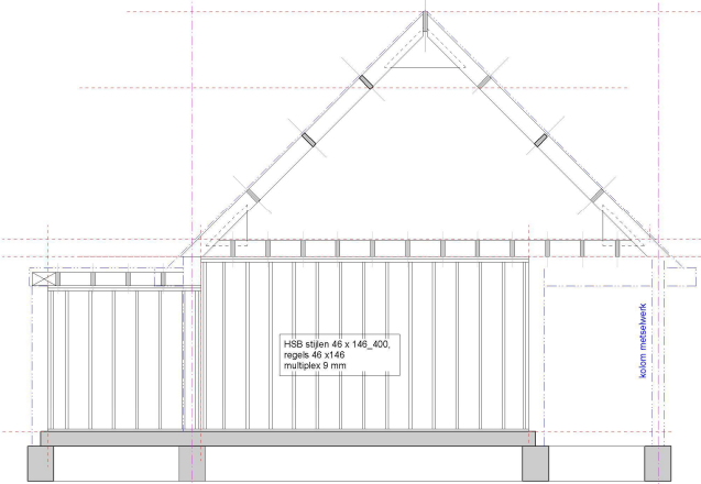
Wandaanzicht E
