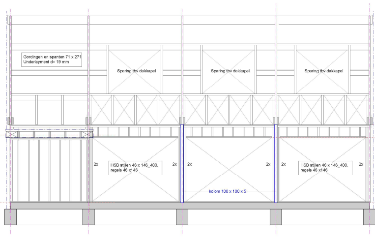
Wandaanzicht G
