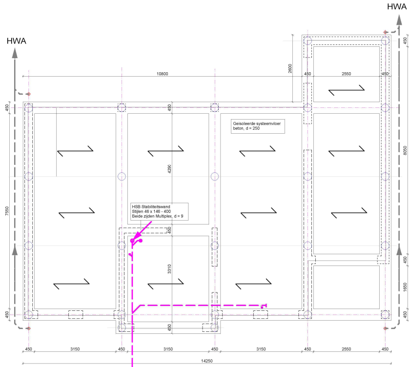
Palenplan
