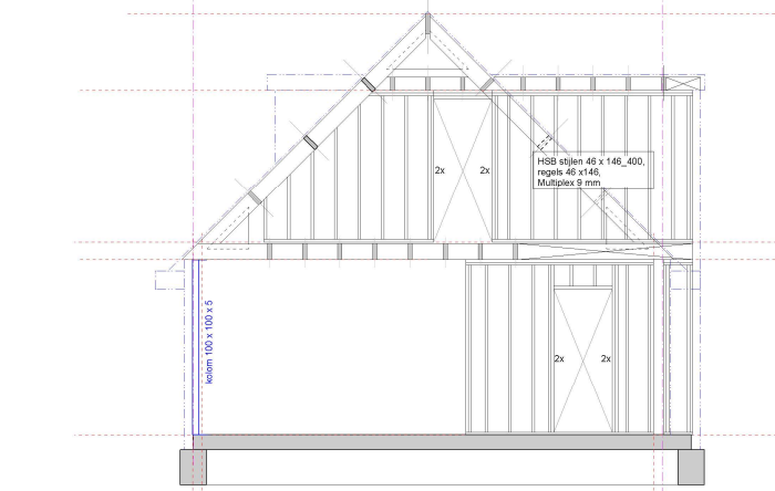
Wandaanzicht C
