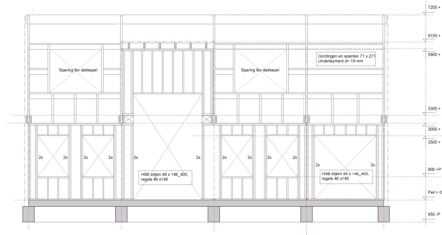
Wandaanzicht F
