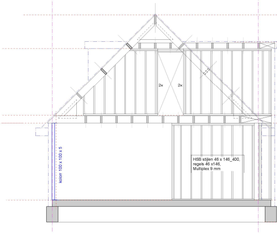
Wandaanzicht B
