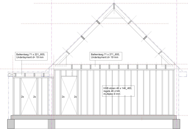
Wandaanzicht D
