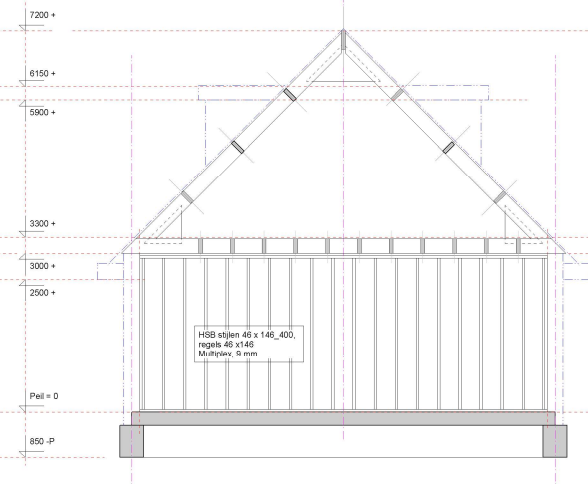
Wandaanzicht A
