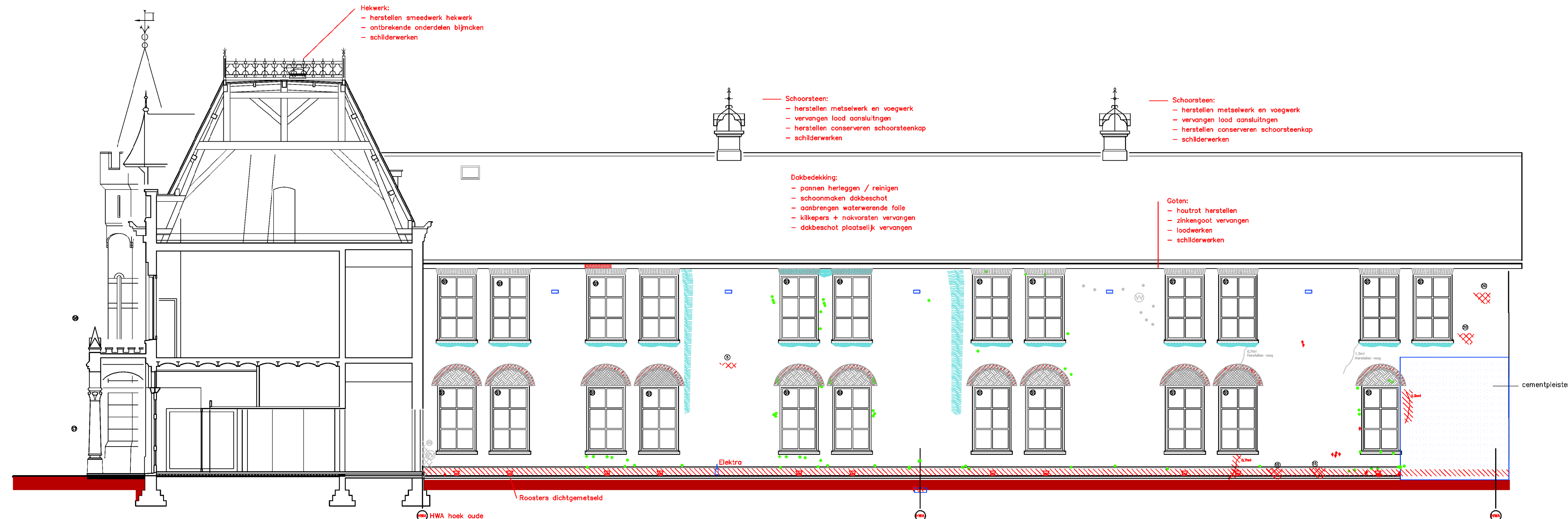
Vleugel 2 Noordgevel
