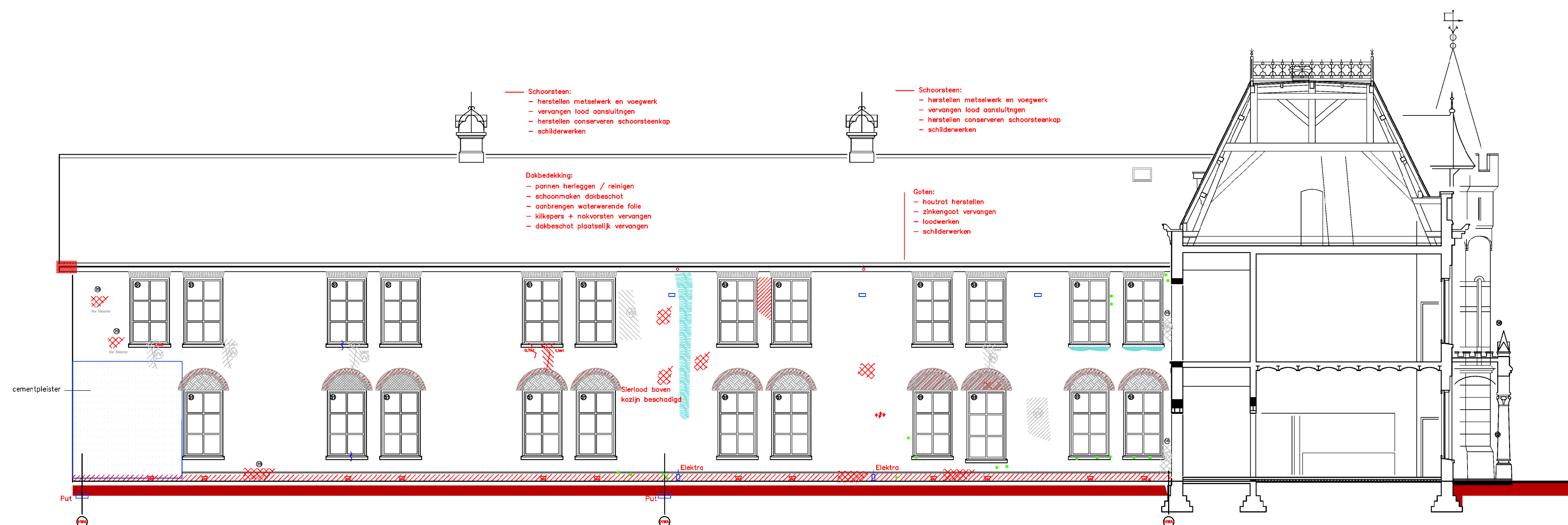
Vleugel 3 Zuidgevel
