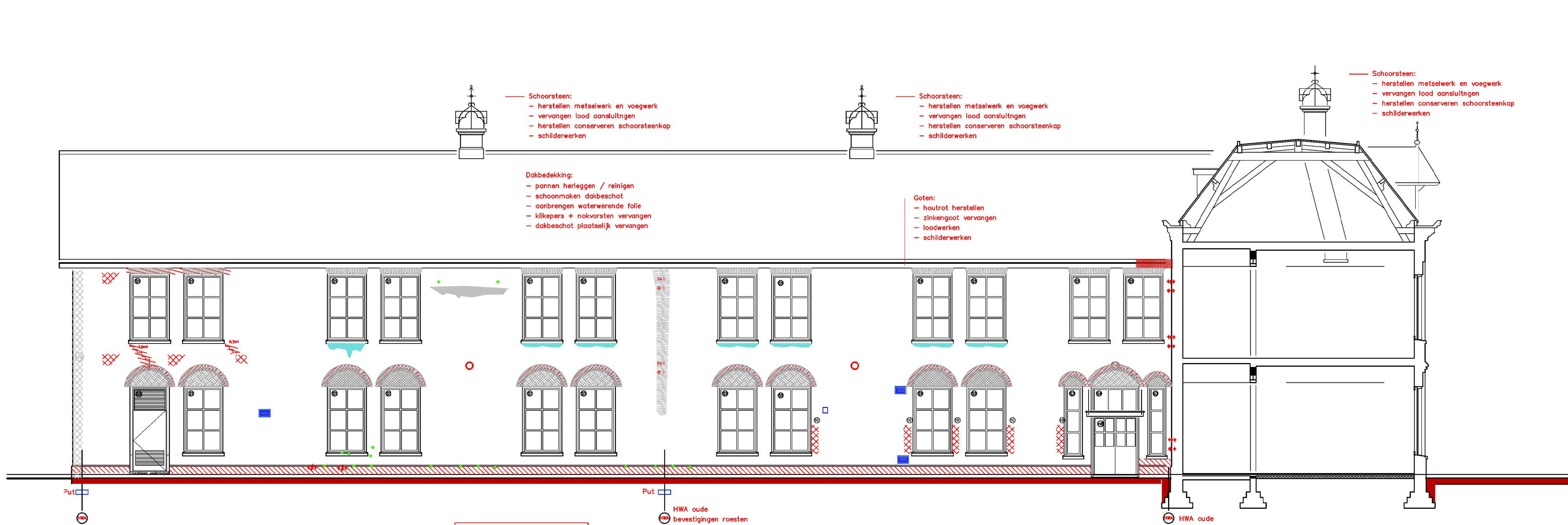
zuidgevel vleugel 4
