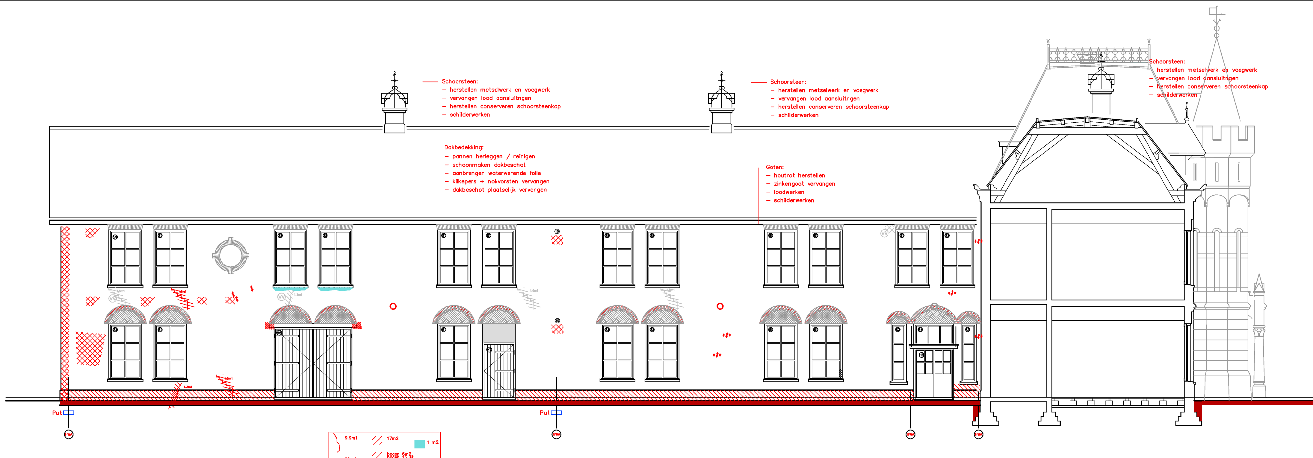
zuidgevel vleugel 2
