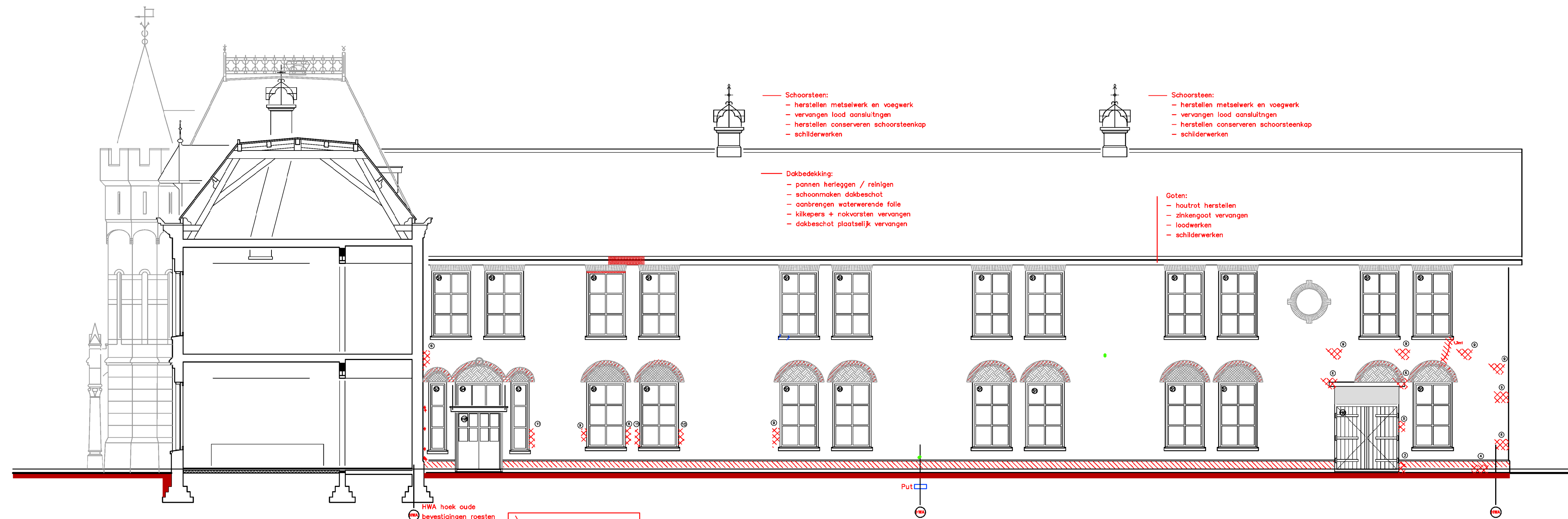
noordgevel vleugel 3
