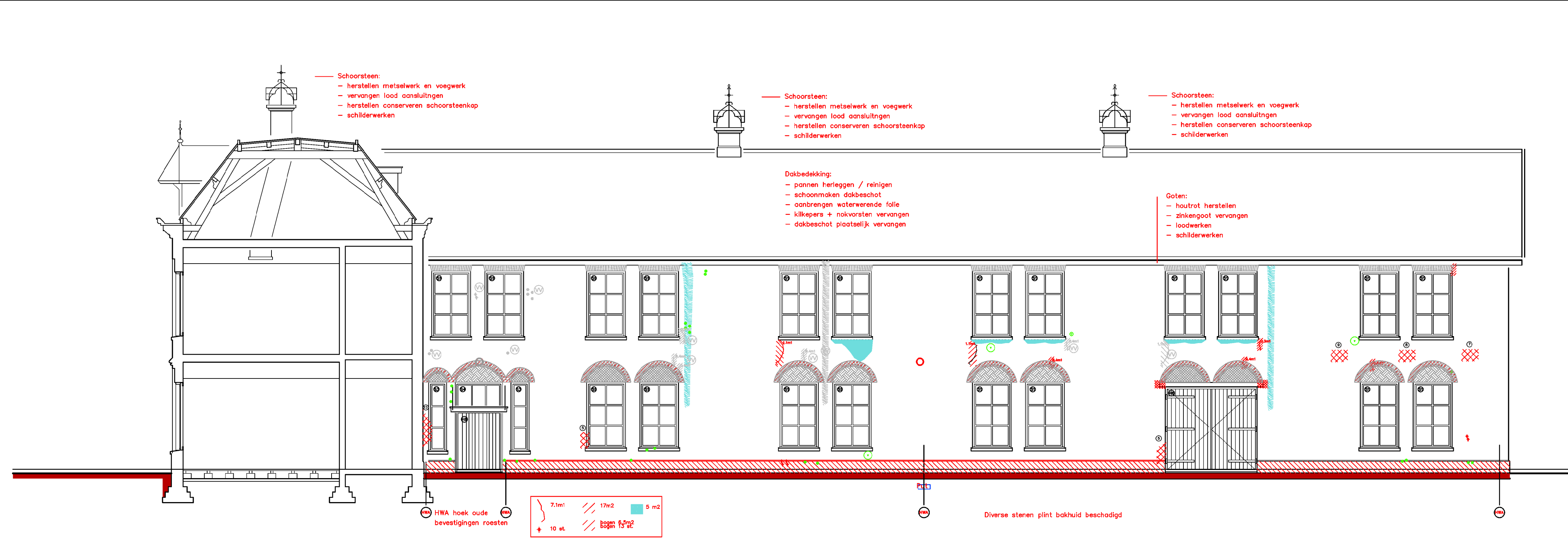
noordgevel vleugel 1
